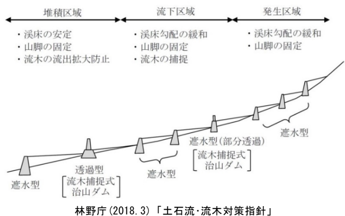
図 1 治山施設の配置例(流木対策)
