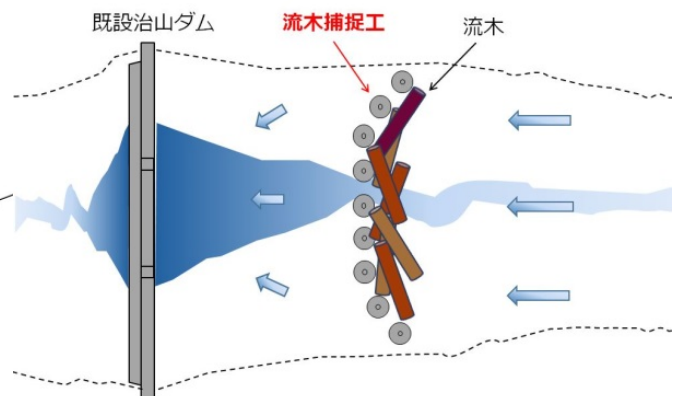
図5 流木捕捉工の配置位置(平面図)
