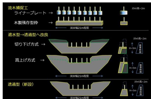
図8 コスト比較する各種透過型治山ダム等
