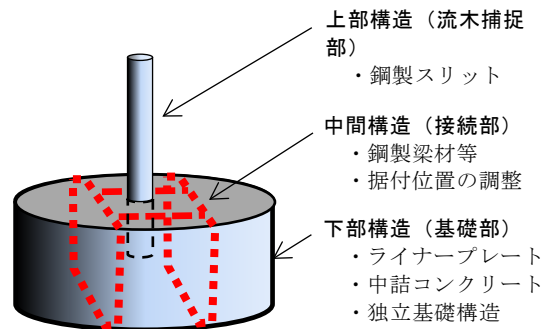
図3 流木捕捉工の構造概要
