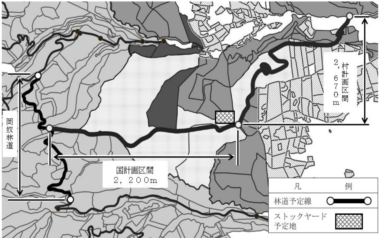
図 4 林道新設ルート
