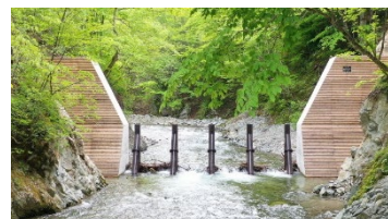
流木捕捉式治山ダムの設置
