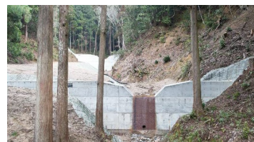
土砂流出を防止する治山ダム群の整備
