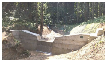
土砂流出を防止する治山ダム群の整備
