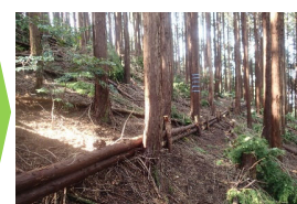
保安林整備（筋工・本数調整伐）
