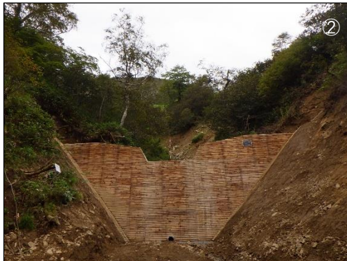
2号コンクリート谷止工
