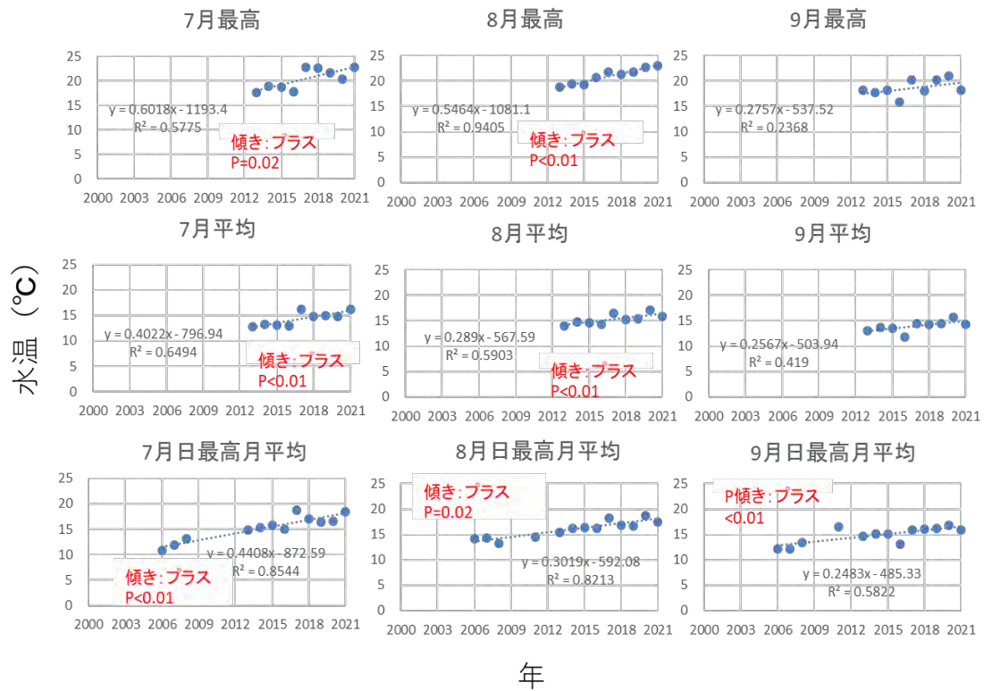
図 9. R3 (2021) 年調査河川・羅臼の 7～9 月の平均水温，日最高水温の平均，最高水温の値の経年変化
