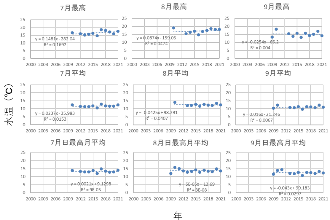
図 10. R3 (2021) 年調査河川・ポン春茹古丹の 7～9 月の平均水温，日最高水温の平均，最高水温の値の経年変化
