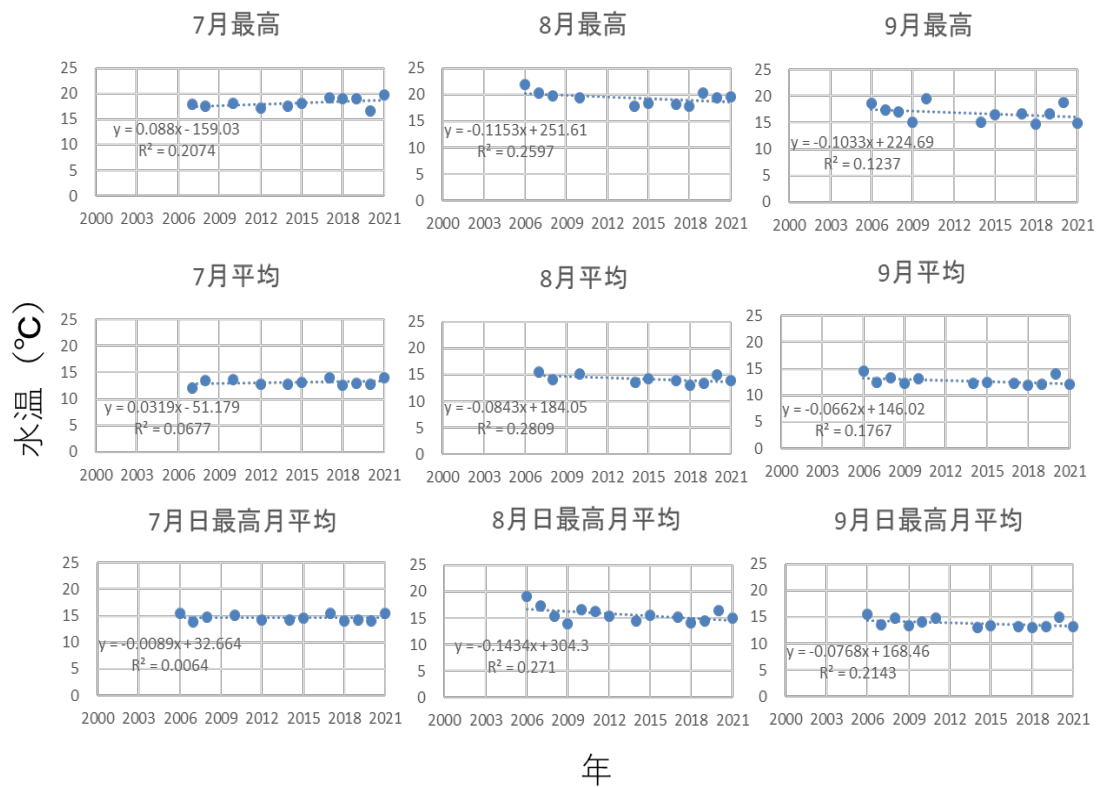
図 5. R3 (2021) 年調査河川・アイドマリの 7～9 月の平均水温，日最高水温の平均，最高水温の値の経年変化
