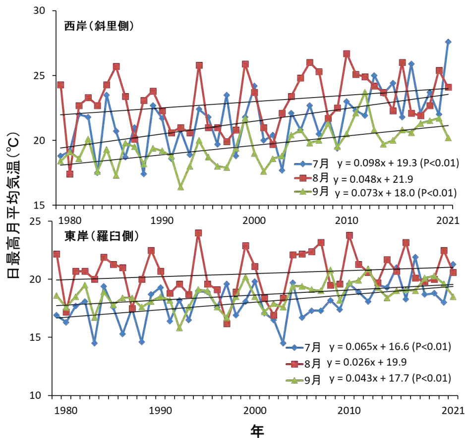
図 27. 西岸（斜里町側）と東岸（羅臼町側）における 7～9 月の日最高月平均気温の経年変化
