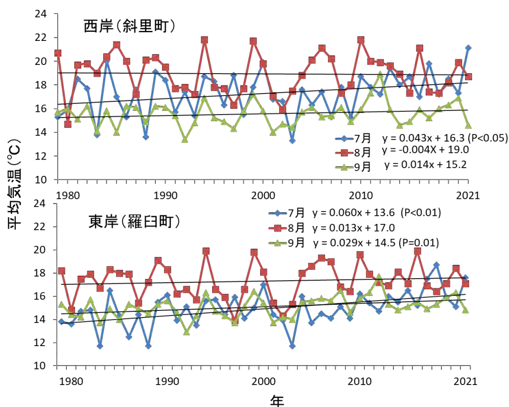
図 25. 西岸（斜里側）と東岸（羅臼側）における7～9月の平均気温の経年変化
