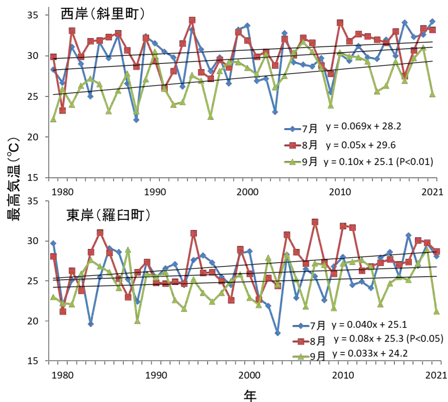
図 26. 西岸（斜里町側）と東岸（羅臼町側）における 7～9 月の最高気温の経年変化
