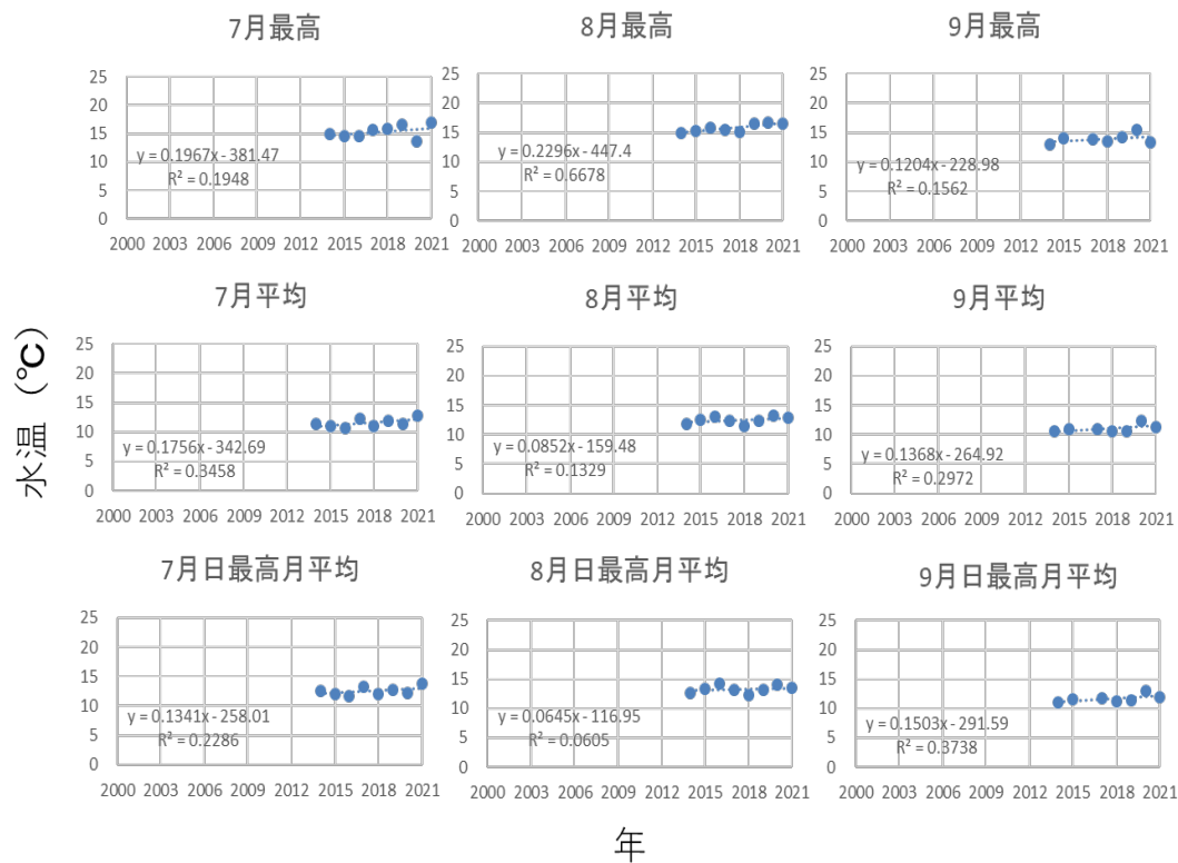
図 4. R3（2021）年調査河川・モイレウシの 7～9 月の月最高，月平均，日最高月平均，それぞれの水温の経年変化
