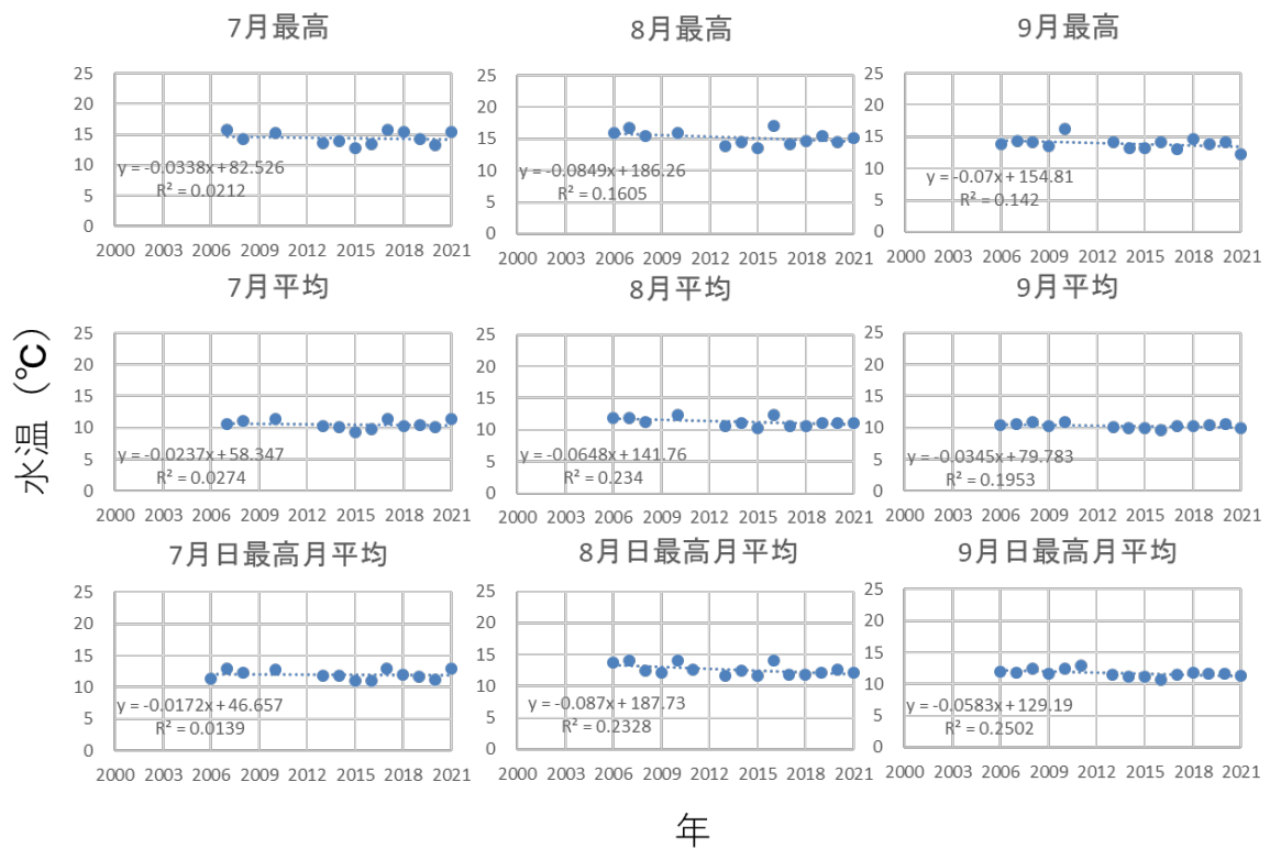
図 6. R3 (2021) 年調査河川・ケンネベツの 7～9 月の平均水温，日最高水温の平均，最高水温の値の経年変化
