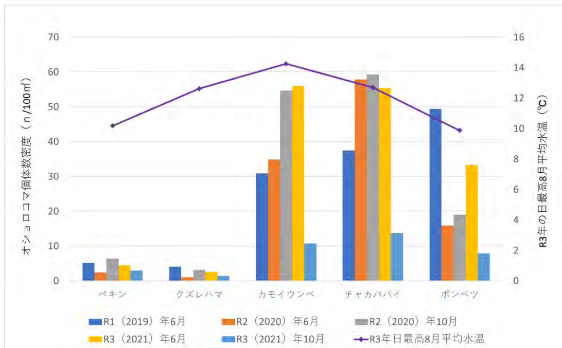
図 14. 半島先端 5 河川のオショロコマ個体数密度と水温の関係
