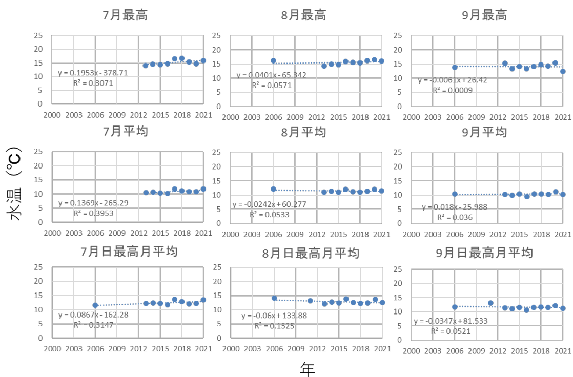
図 8. R3 (2021) 年調査河川・サシルイの 7～9 月の平均水温，日最高水温の平均，最高水温の値の経年変化
