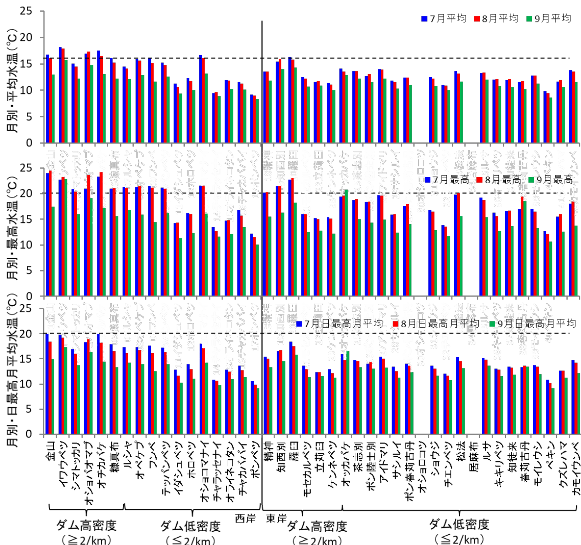
図3. R3（2021）年の7～9月に観測された月毎の日平均水温の平均、日最高水温の平均および日最高月平均水温
