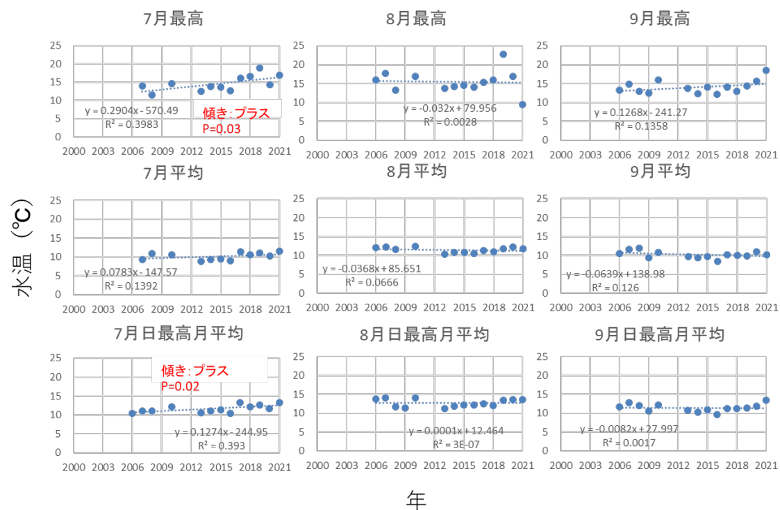
図 11. R3 (2021) 年調査河川・春荻古丹の 7～9 月の平均水温，日最高水温の平均，最高水温の値の経年変化.
