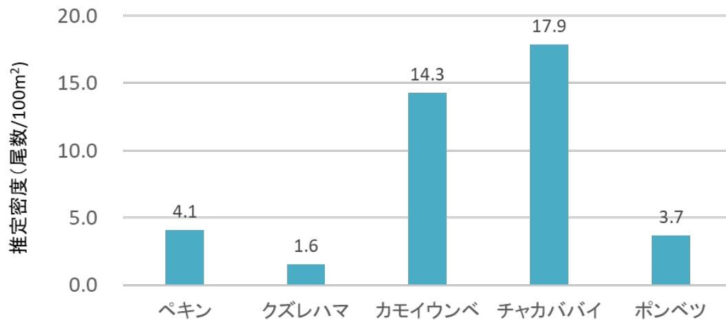
図 19. qPCR 法によるオショロコマ推定生息密度（尾数/100 m 2 ）
