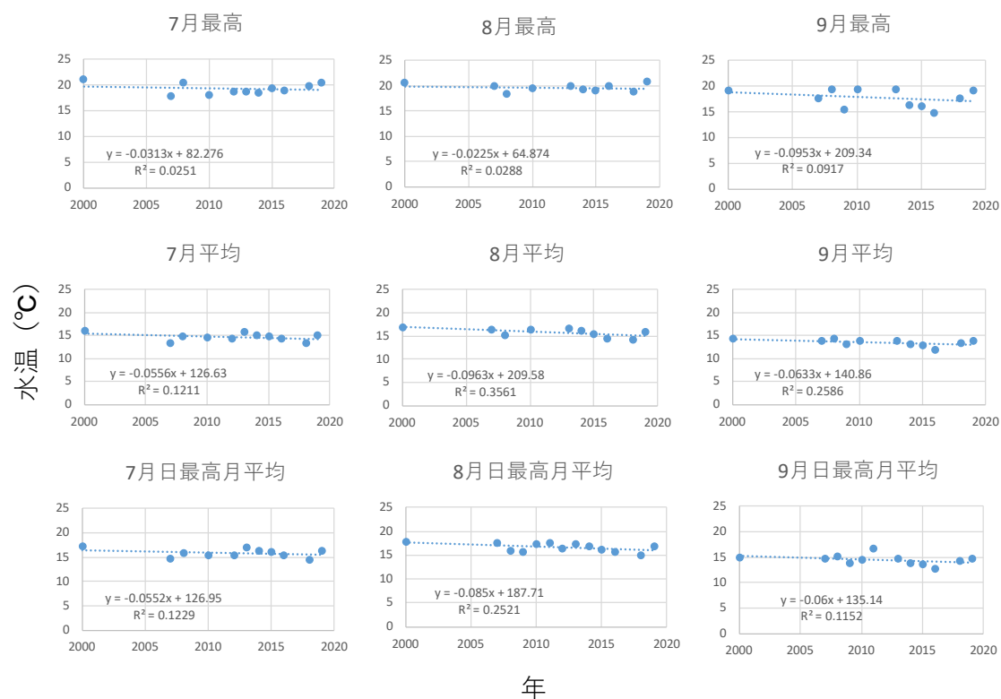
図 5. R1 (2019) 年調査河川・オショコマナイの 7～9 月の平均水温，日最高水温の平均，最高水温の値の経年変化
