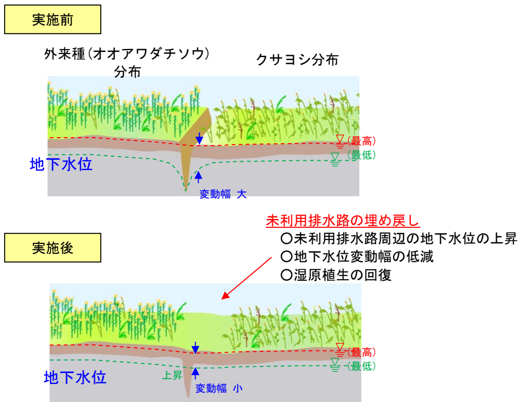
図 4-7(1) 未利用排水路埋め戻しのイメージ(A区域)
