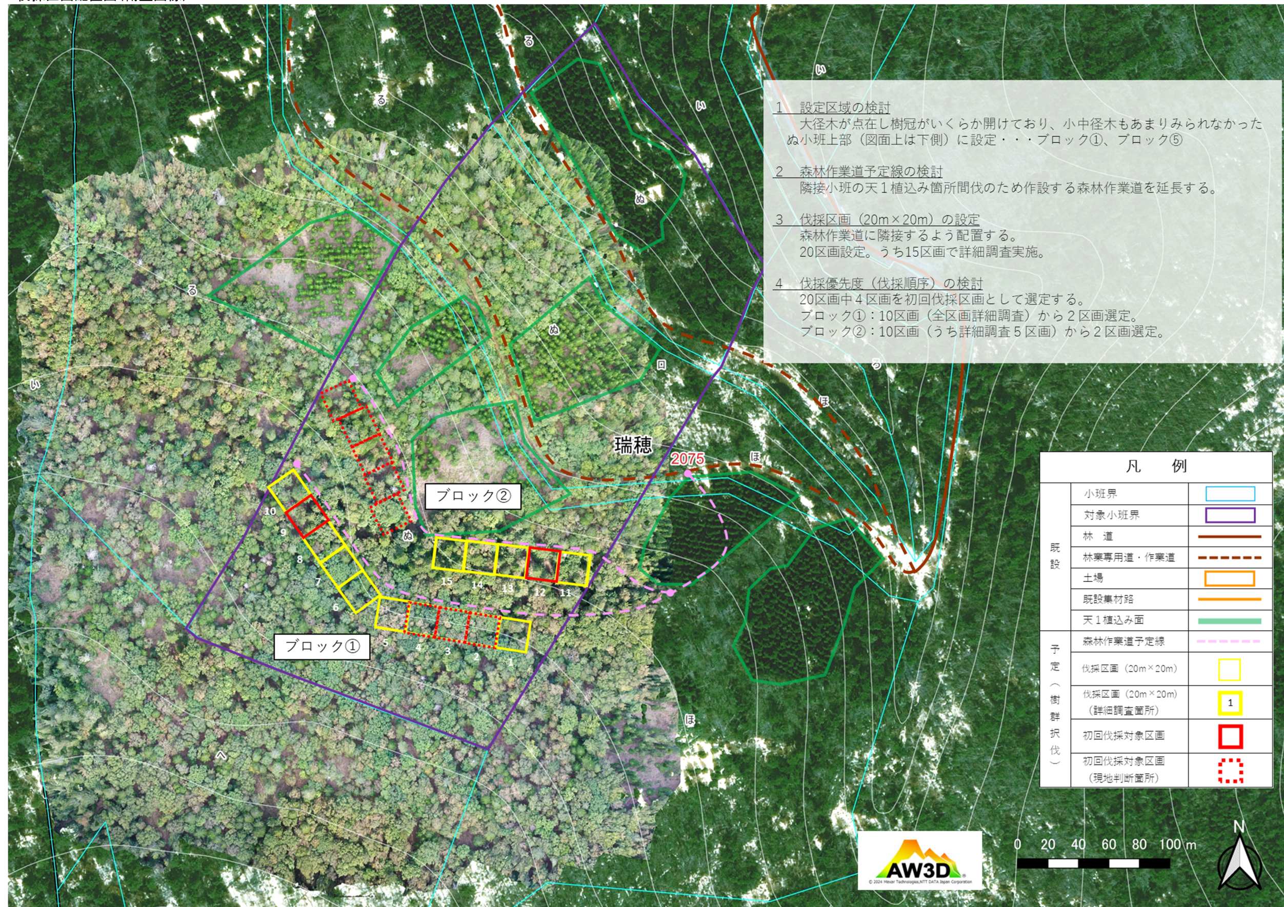
図 3.4.5 伐採区画配置図(瑞穂)
