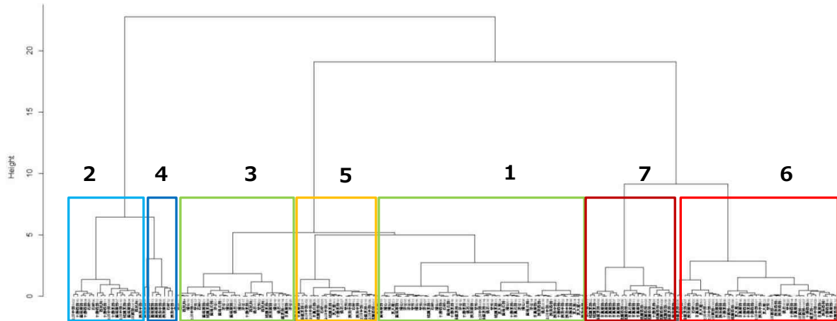
図-3.3.39 クラスタ結果のデンドログラム
