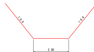
水路工断面図 S=1:50
