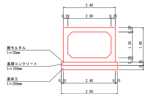
ボックスカルパート工標準図 S=1:50
