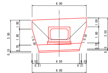
吐口正面图 S=1:100
