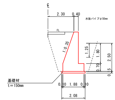
吐口側面図 S=1:100
