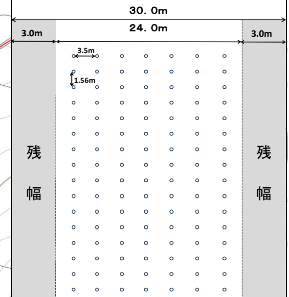
429ほ地拵・植付型式詳細図(7条植栽)
