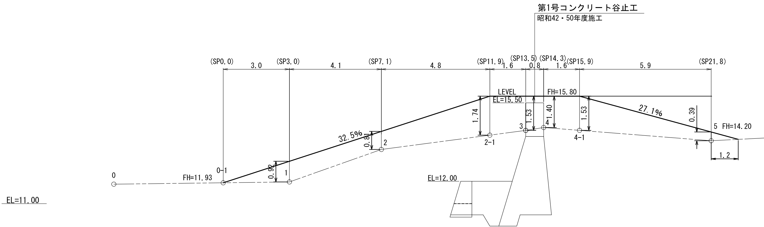
側 面 図
