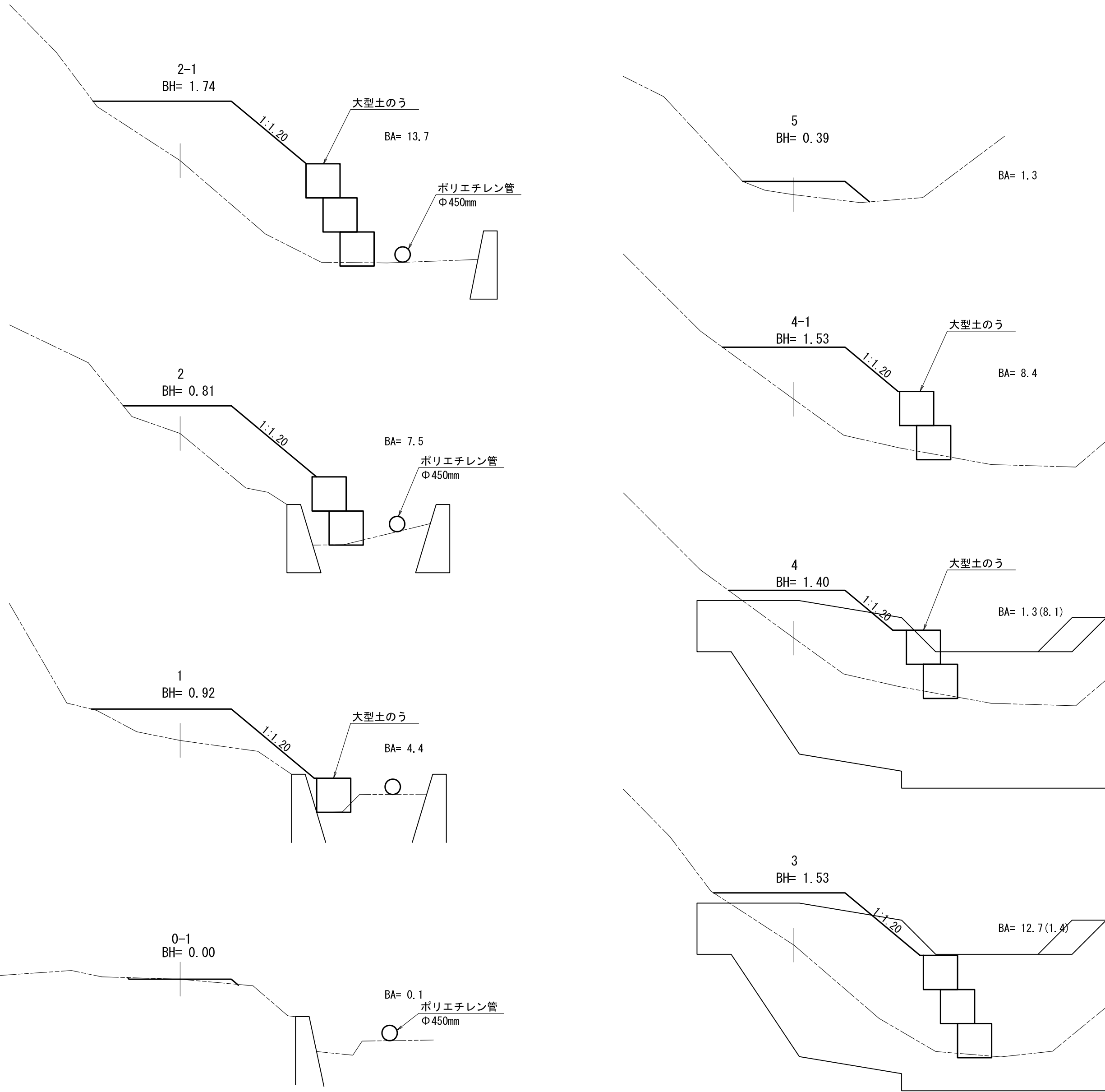
横 断 図
