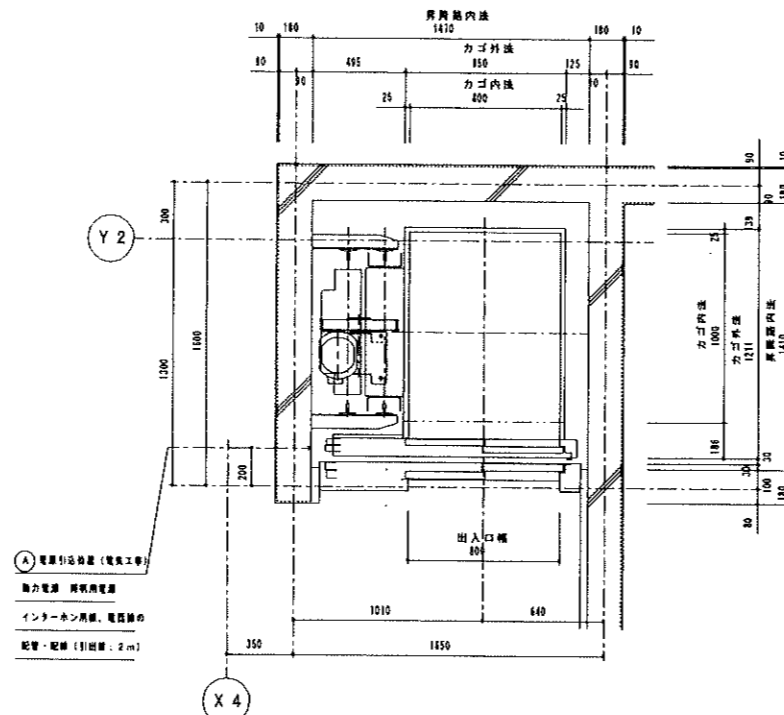
昇降路平面図 (1/20)
