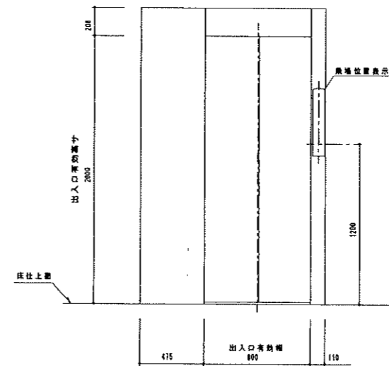
乗場正面図 (1/20)
