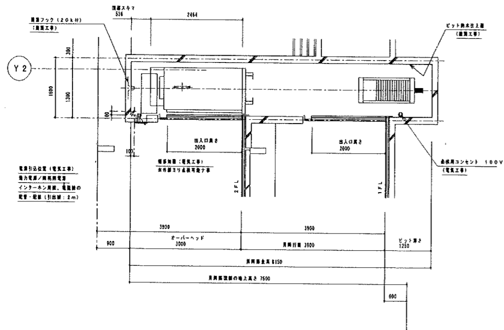
昇降路縦断面図 (1/50)
