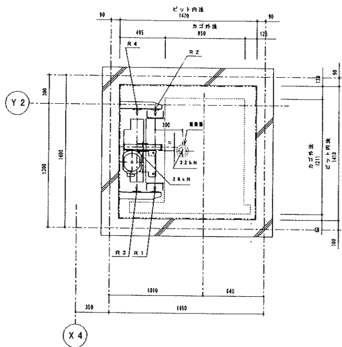
ピット平面図 (1/20)
