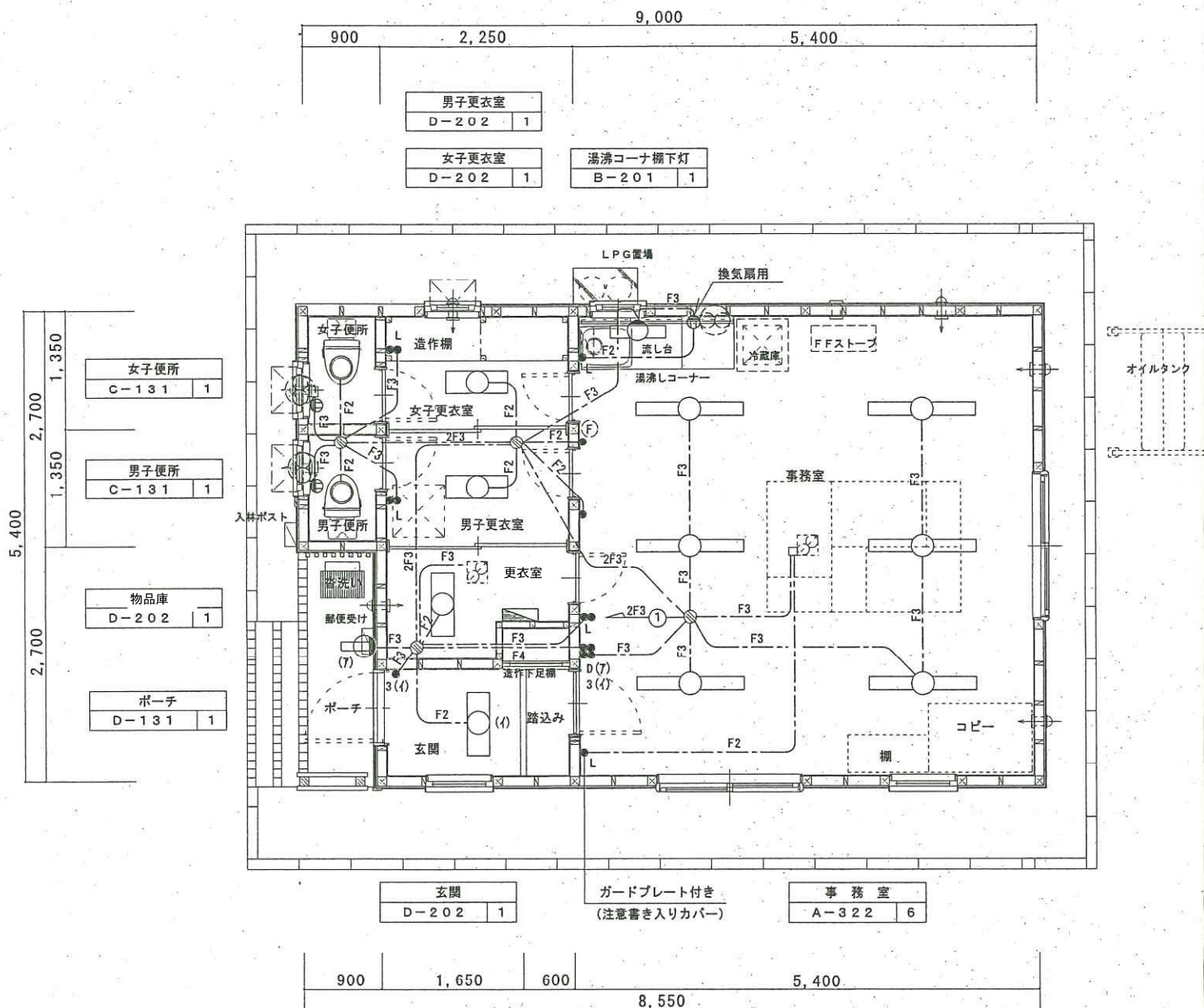
平面詳細図 S=1/30
