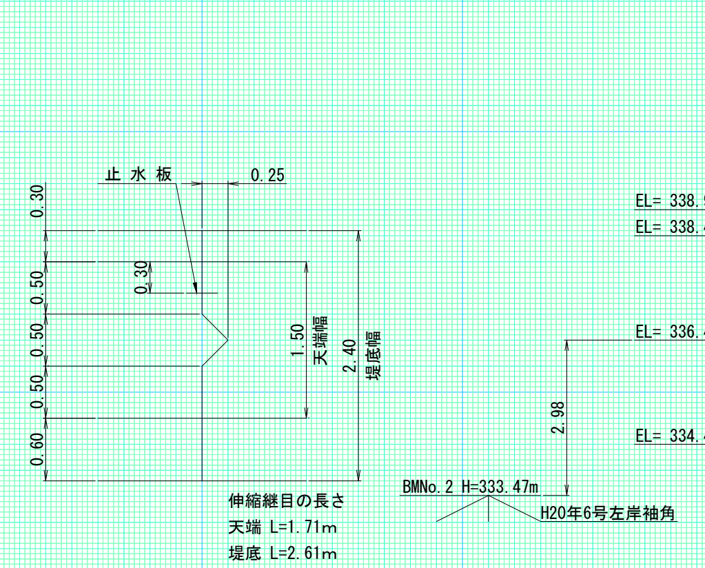
伸縮継目詳細図 S=1:50
