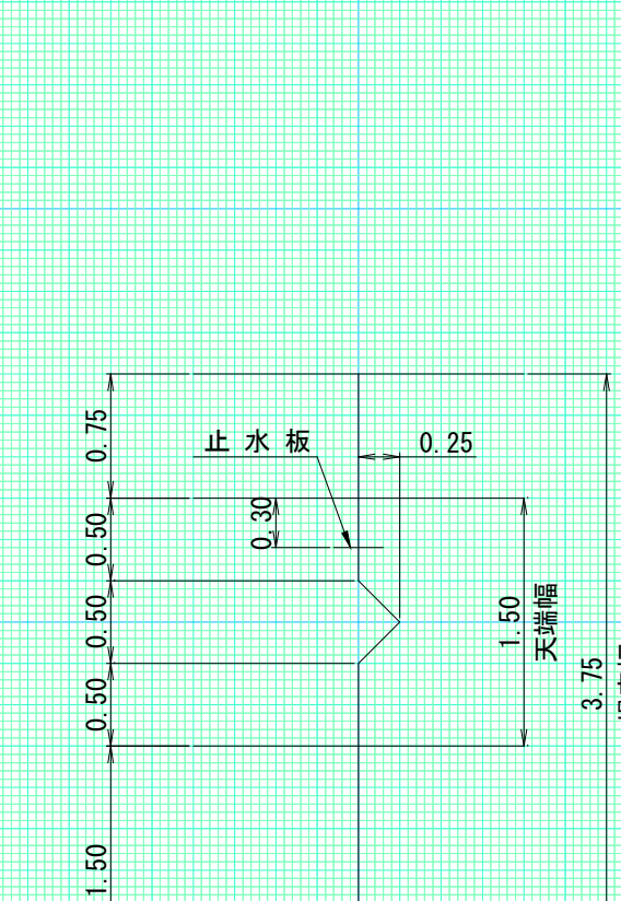
伸縮継目詳細図 S=1:50
