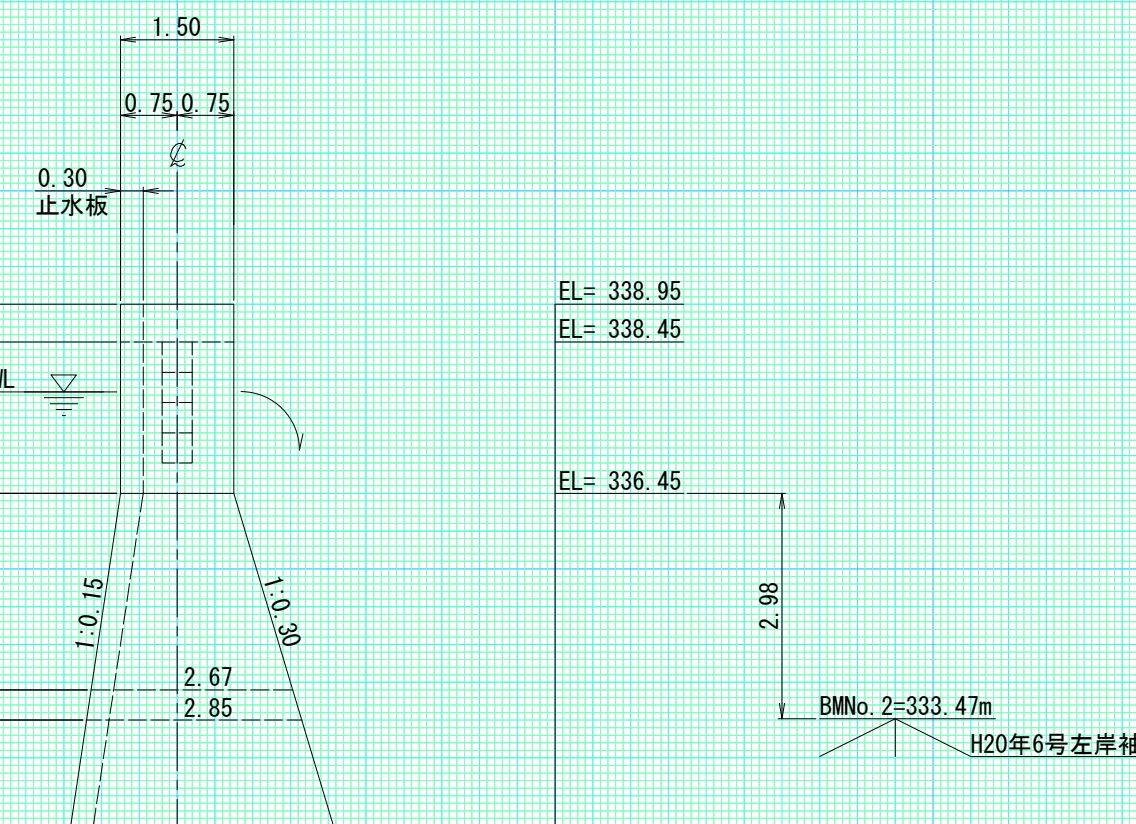
側面図
