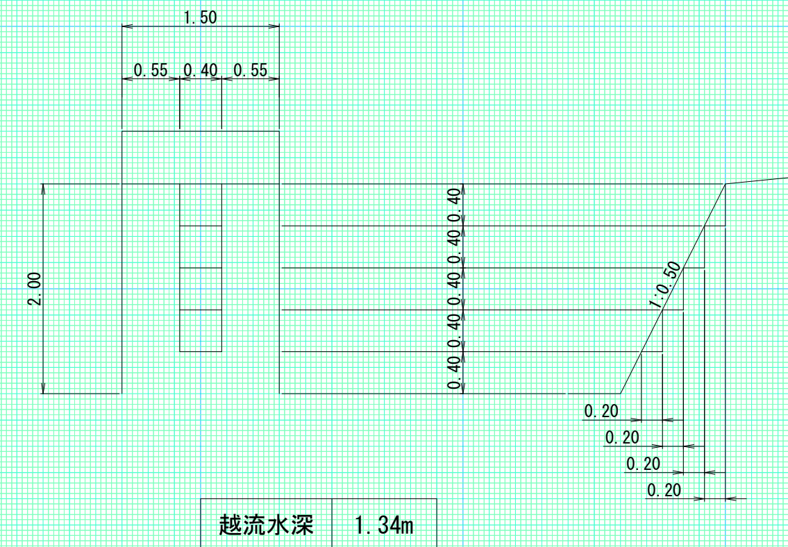
放水路階段詳細図 S=1:50
