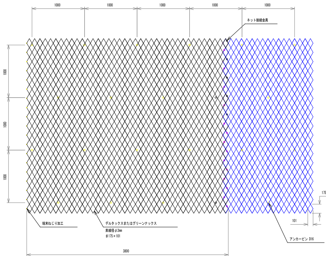
正面図
