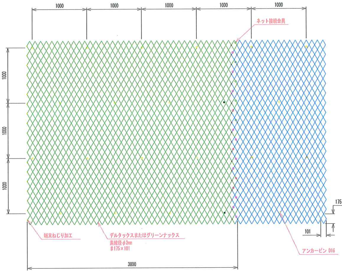
正面図 S=1:30
