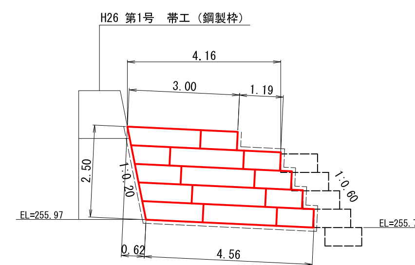
左岸側壁正面図
