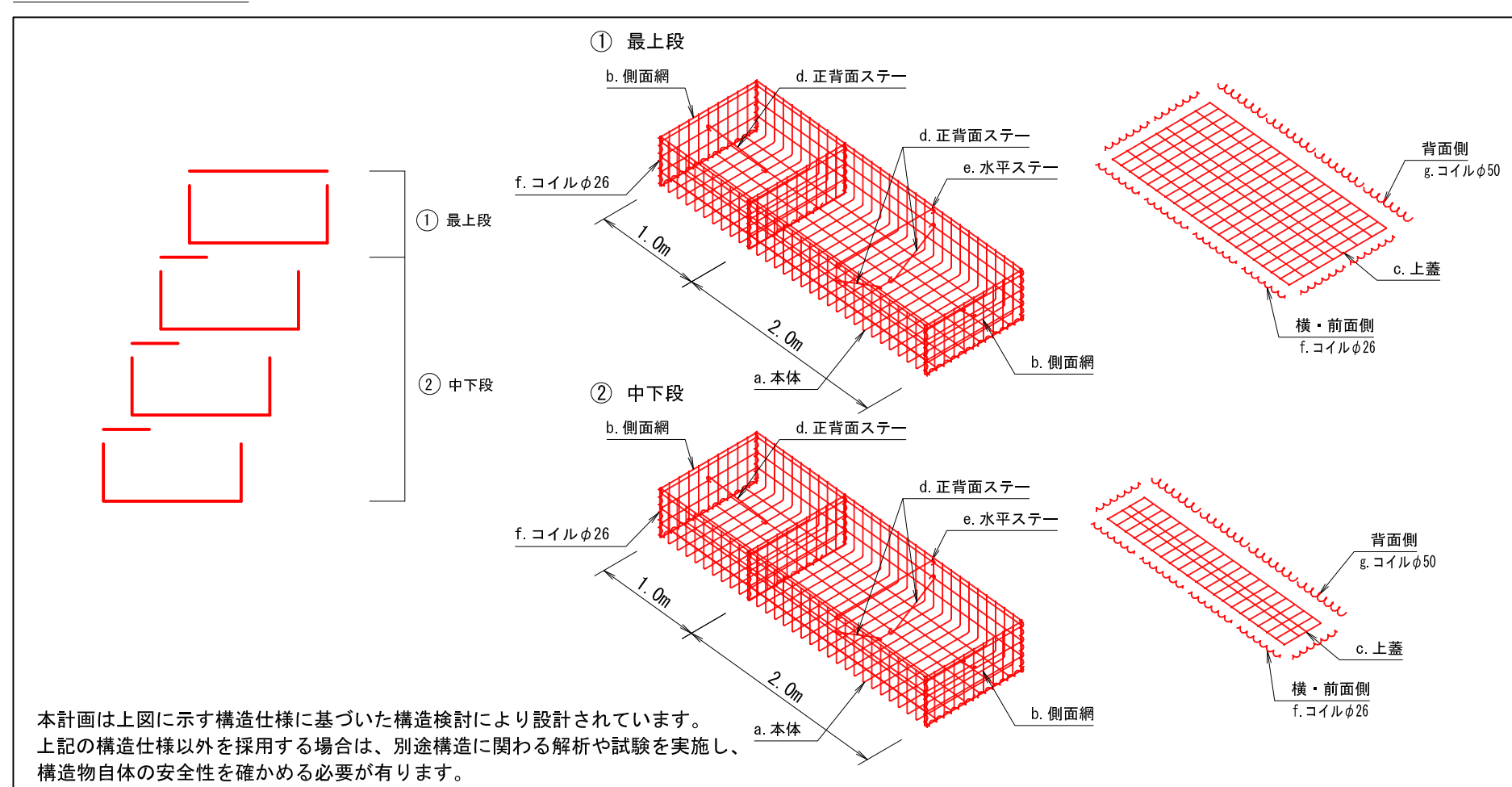
河川用省力化かご工 姿図
