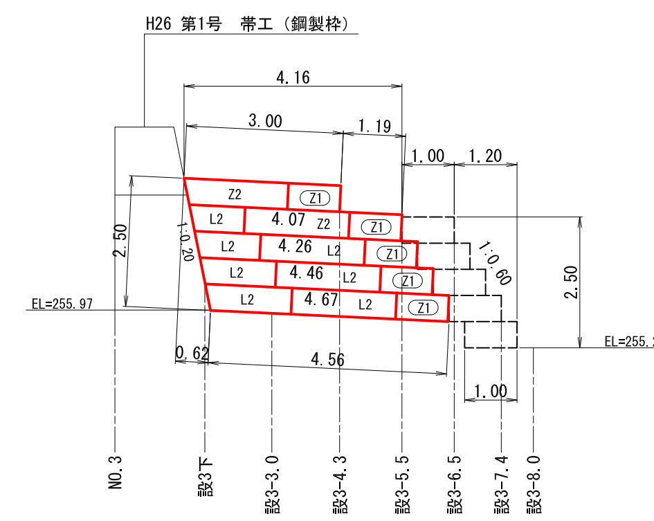
左岸側壁正面図
