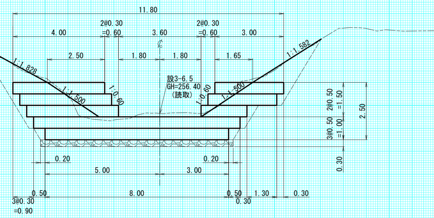
垂直壁正面図
