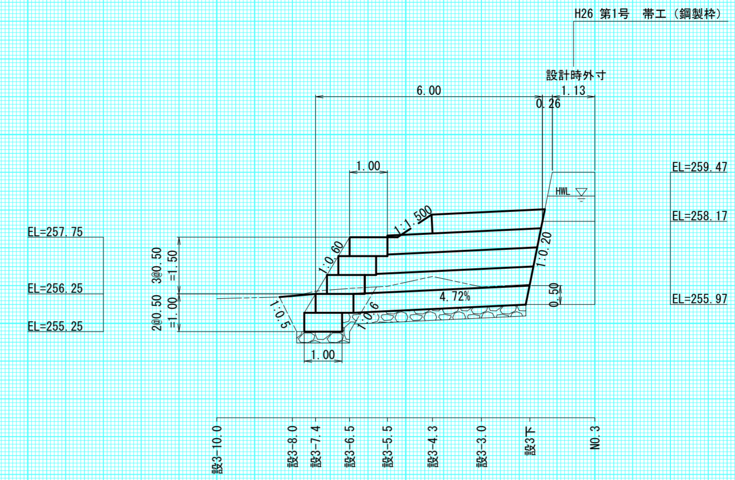
縦断面図
