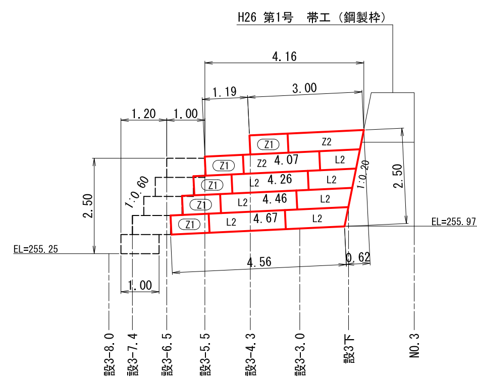
右岸側壁正面図
