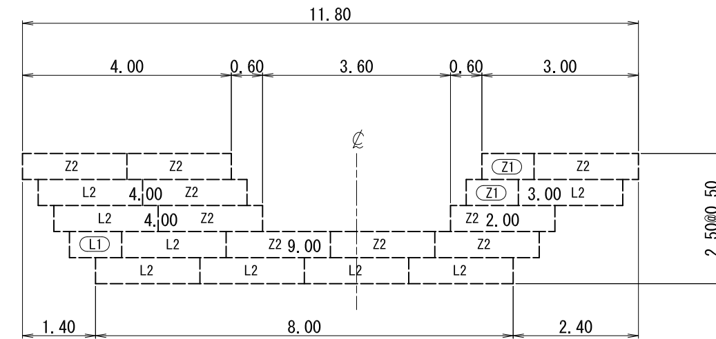
垂直壁正面図
