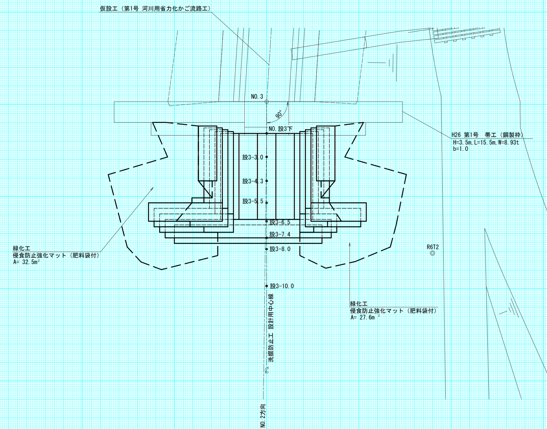
平面図
