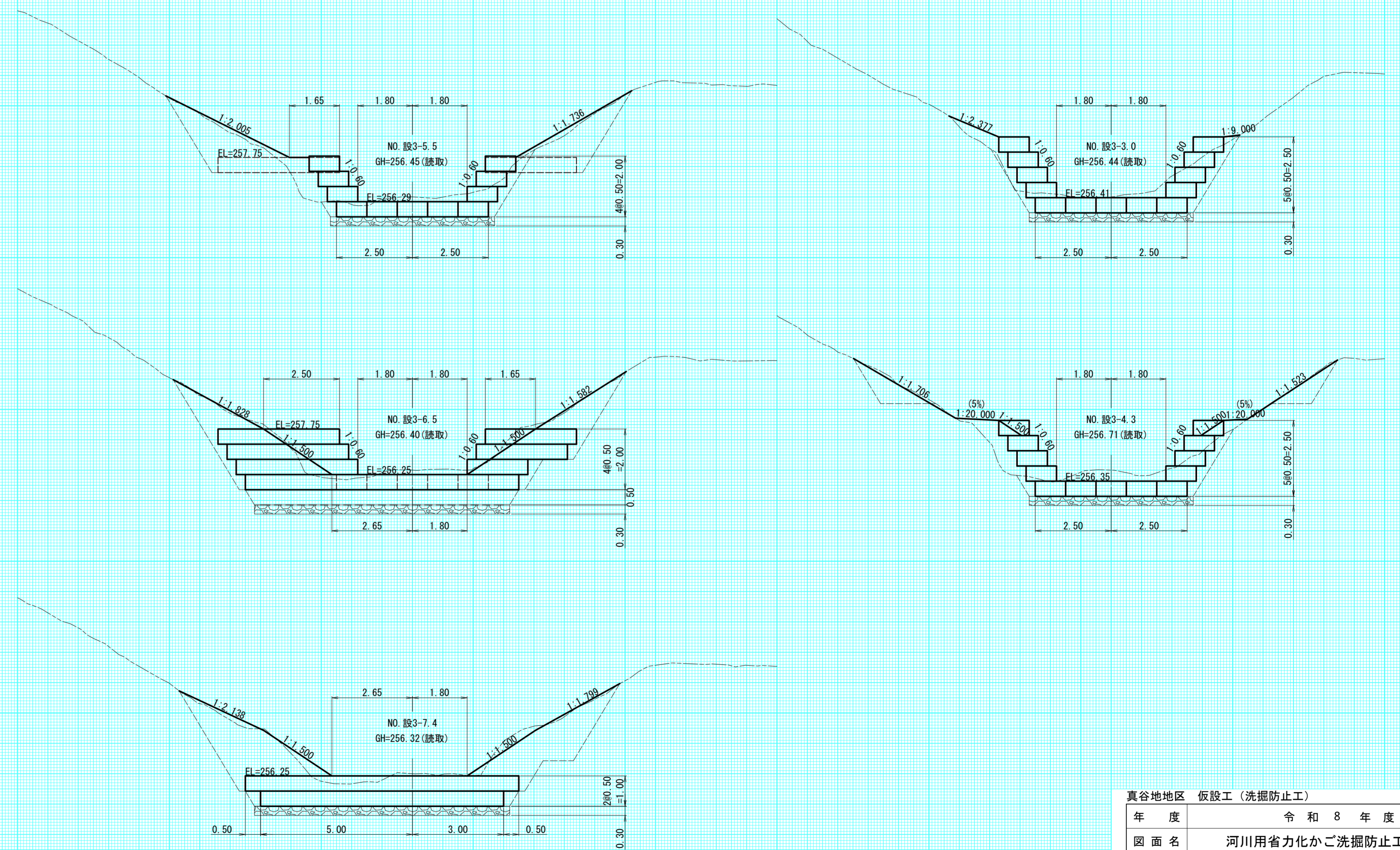
横断面図
