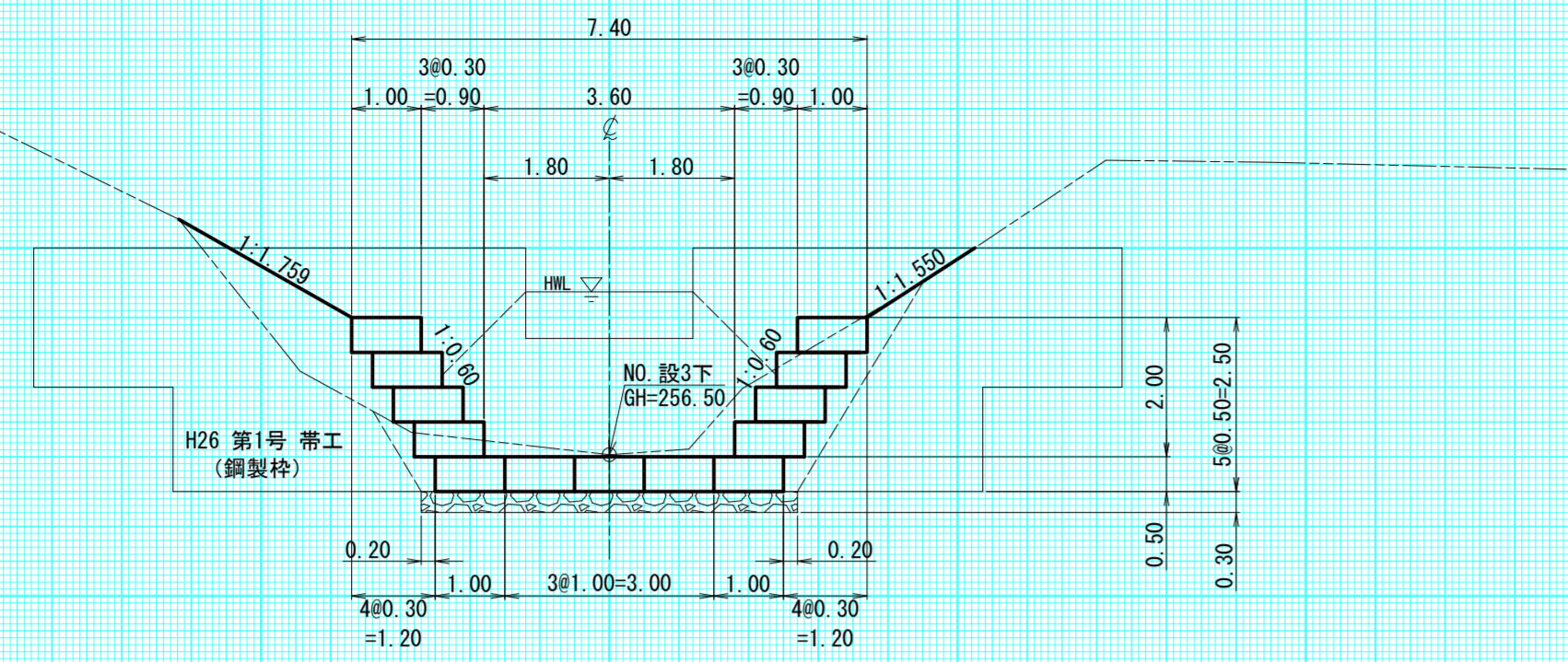
水叩き・流路部 正面図
