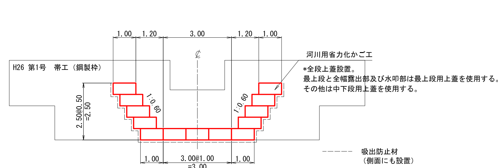
断面図
