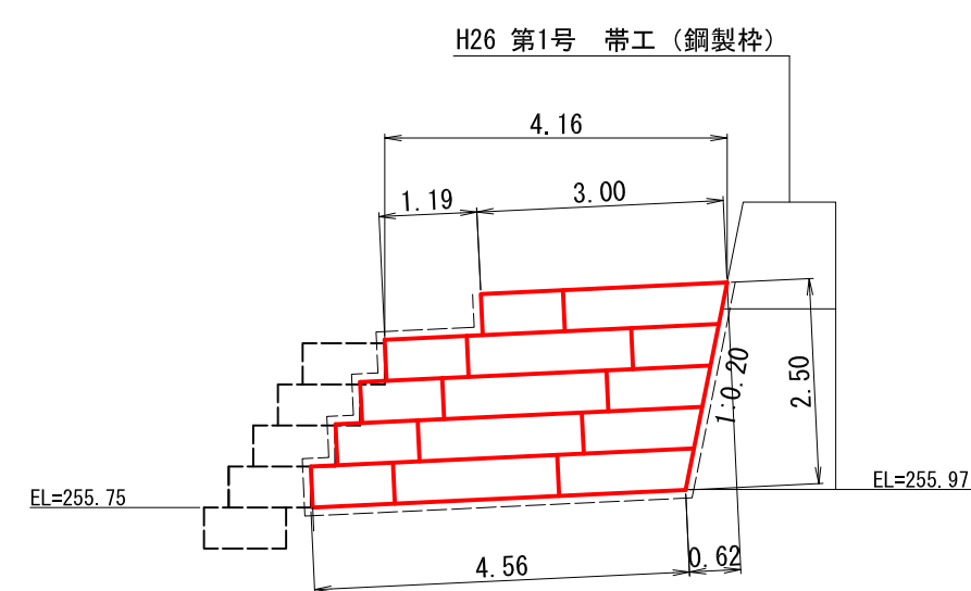
右岸側壁正面図
