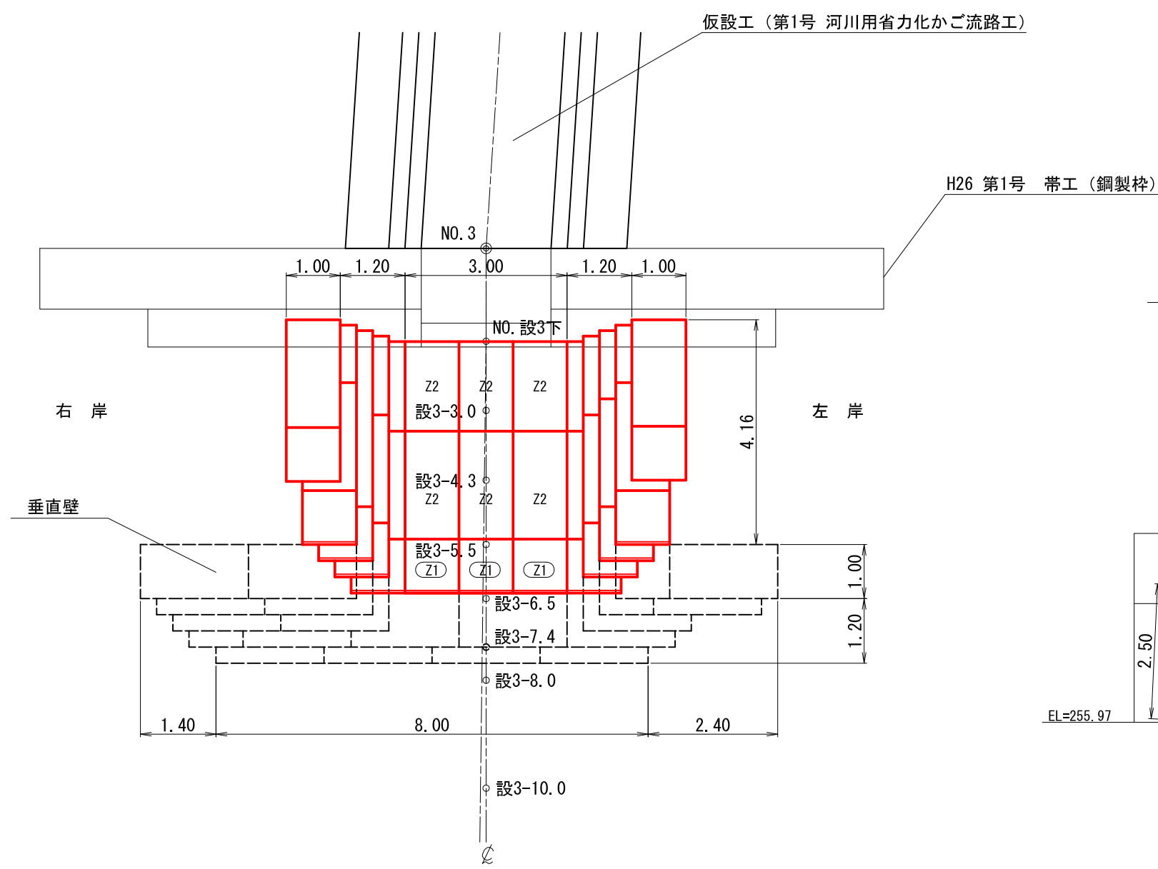
平面図
