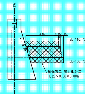
(2号コンクリート谷止工)
