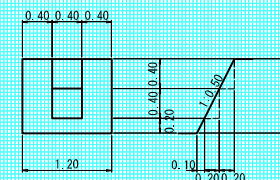
放水路階段詳細図 S=1:50
