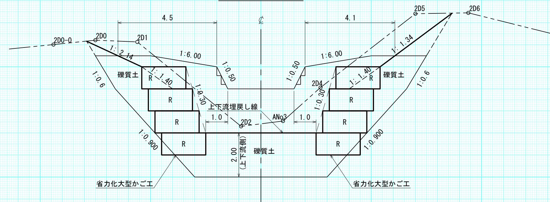
埋戻し図
