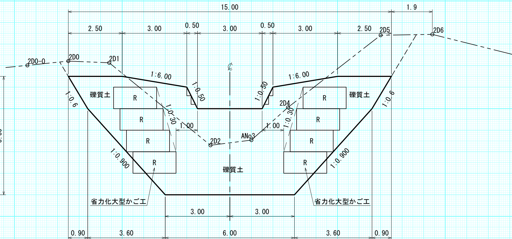
正面図
