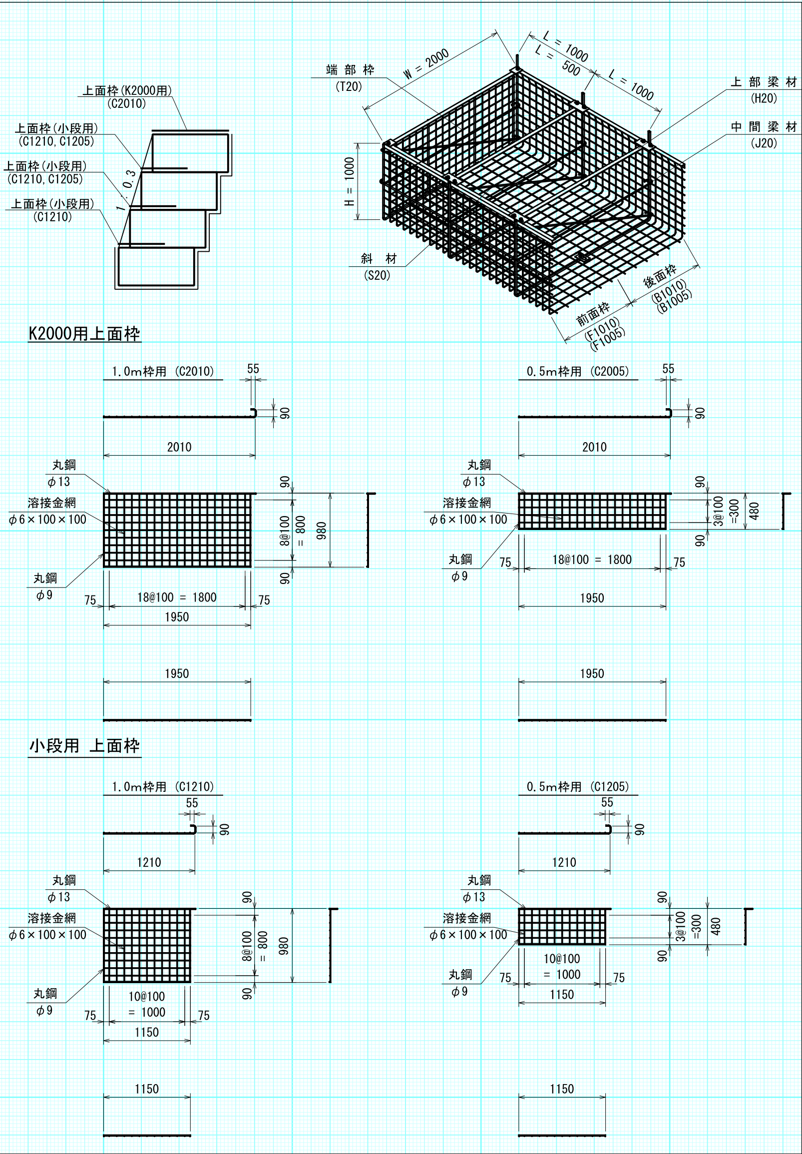
省力化大型かご工 標準図
