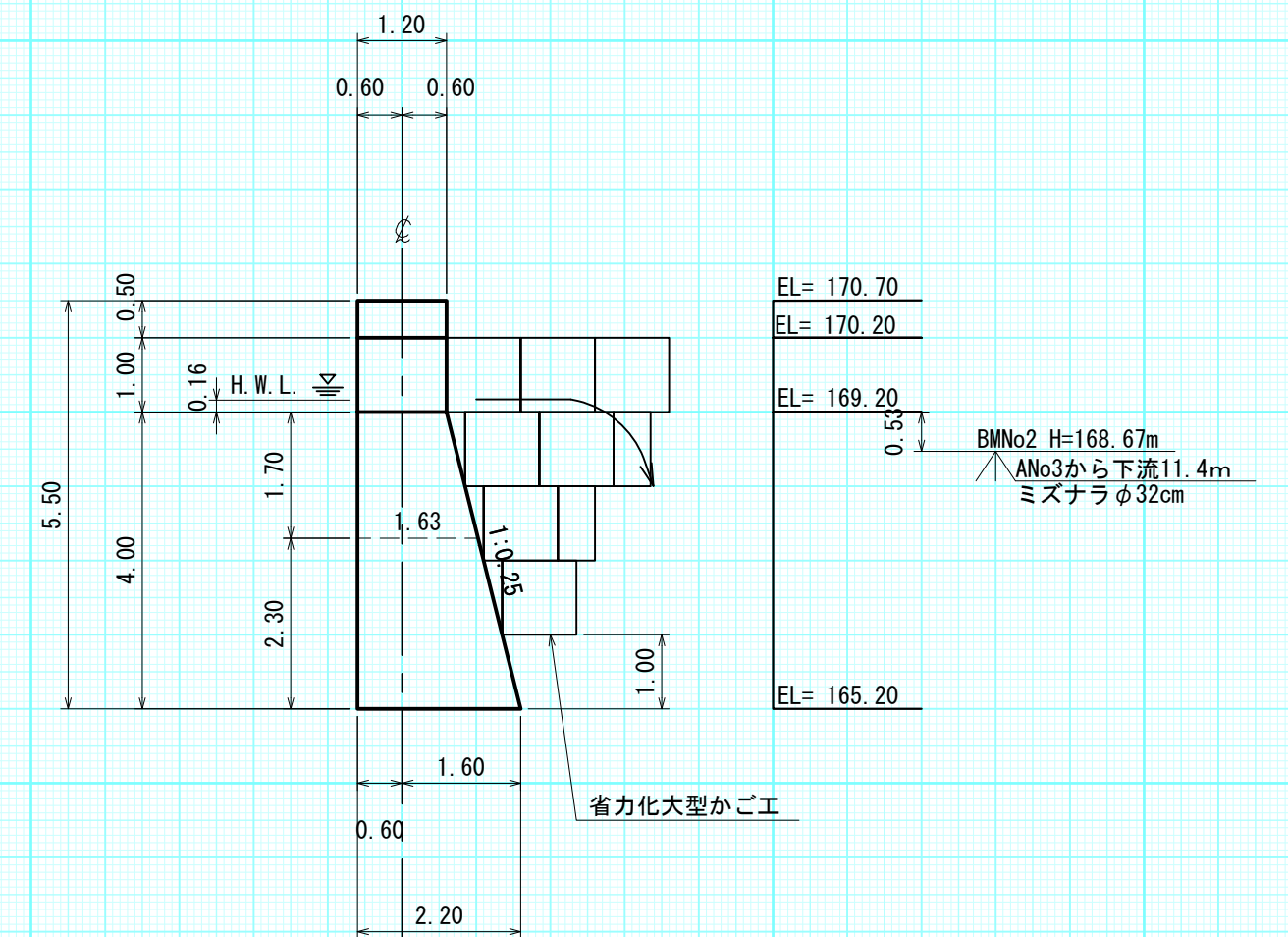
側面図
