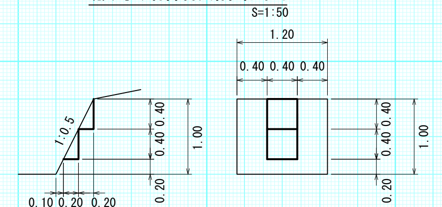
放水路階段詳細図
