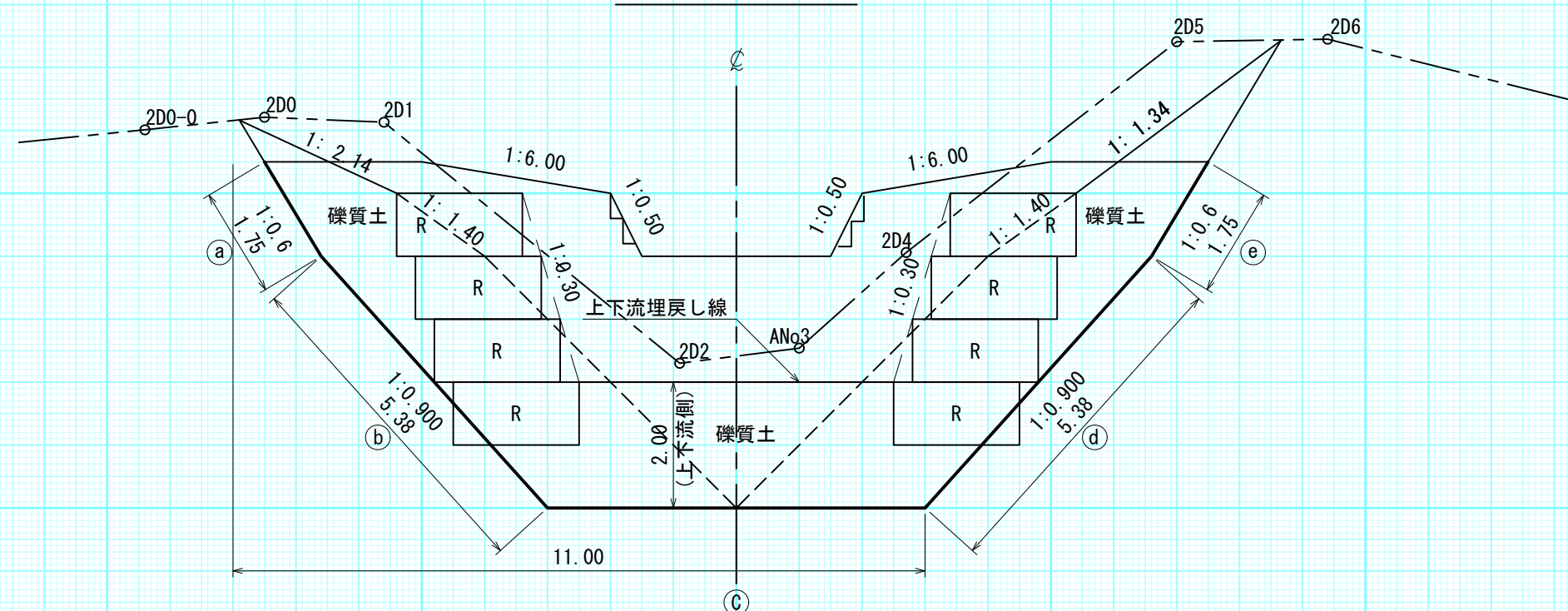
掘削面整形図
