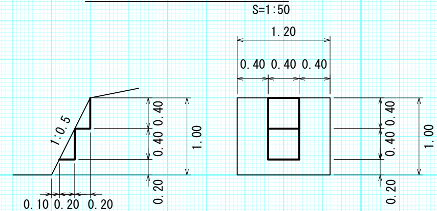
放水路階段詳細図
