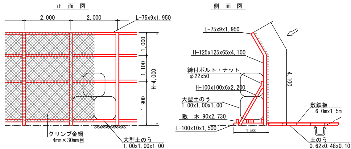
仮設落石防護柵標準図 A1:S=1/ 50 単位:mm A3:S=1/100
