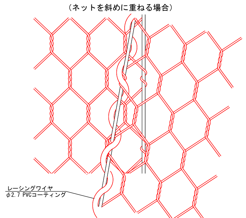
③ ネット連結部詳細図 A1:S=1:3 A3:S=1:6
