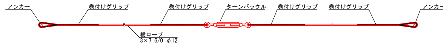
部品詳細図 A1:S=1:3 A3:S=1:6
