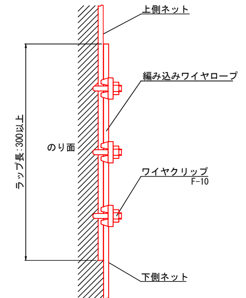
② ネット継ぎ足し部詳細図 A1:S=1:3 A3:S=1:6
