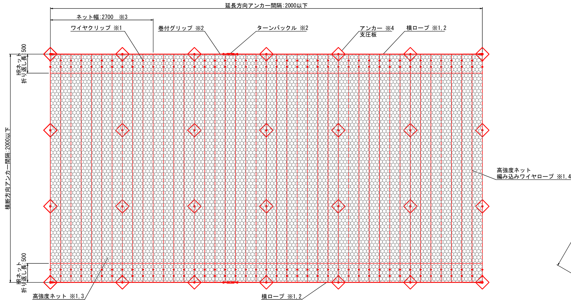
正面図
