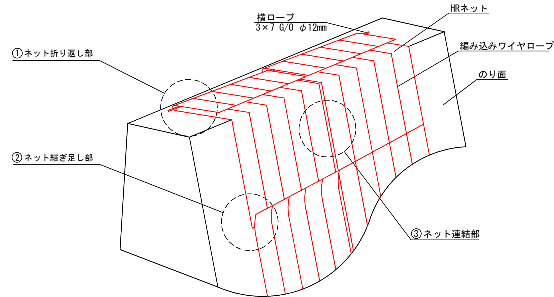
横ロープ取付図 A1:S=1:5 A3:S=1:10
