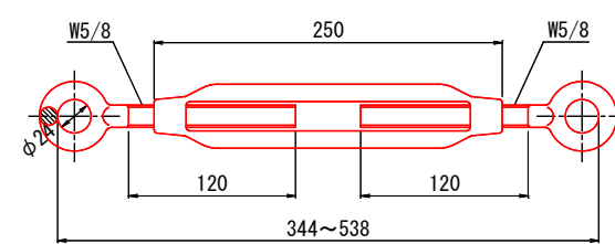
部品詳細図 A1:S=1:3 A3:S=1:6
