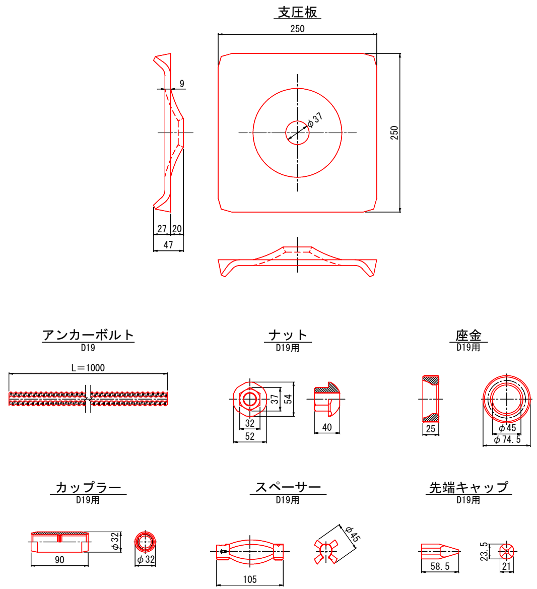
アンカー部品図 A1:S=1:3 A3:S=1:6
