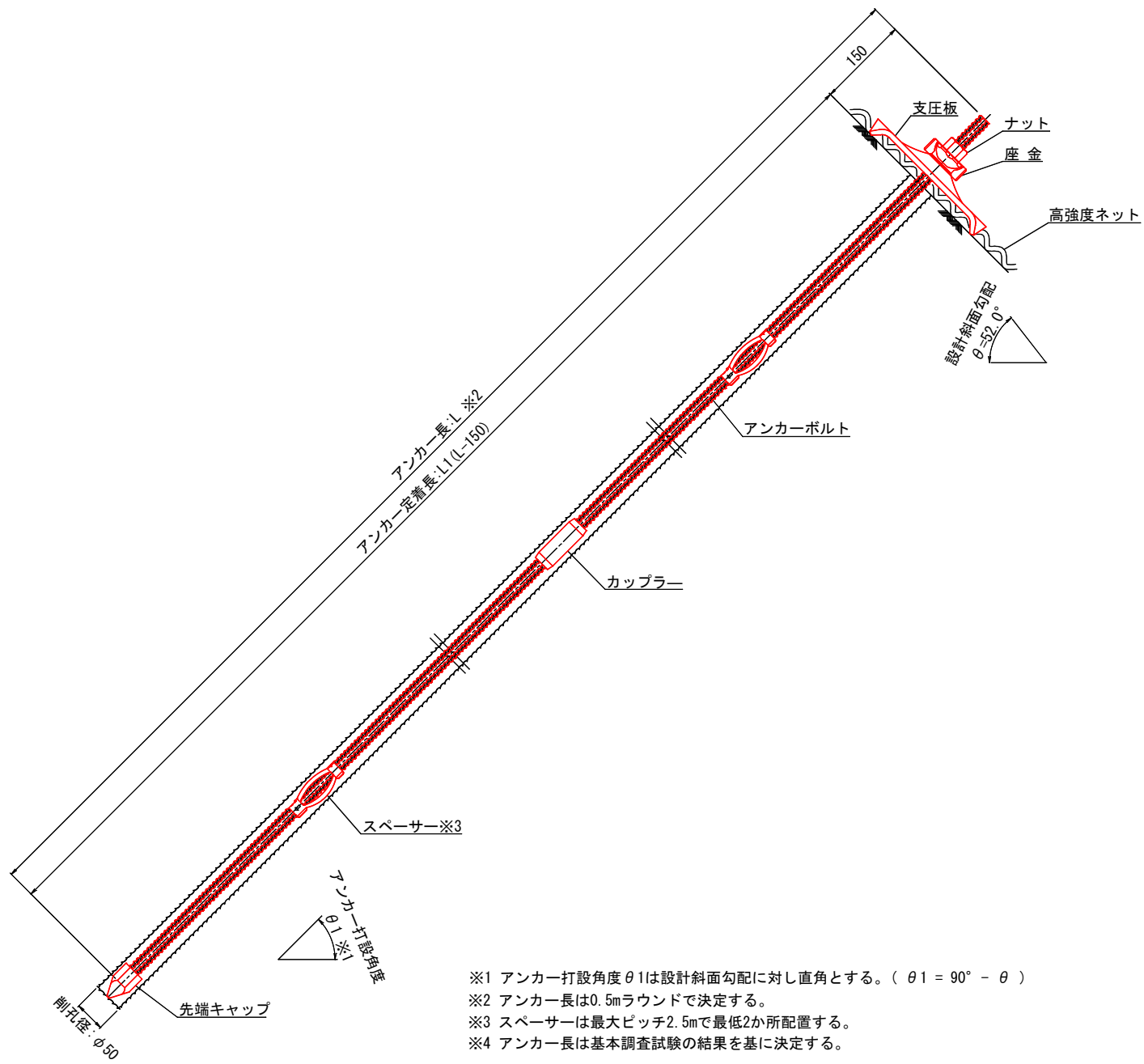
アンカー組立図 A1:S=1: 5 A3:S=1:10
