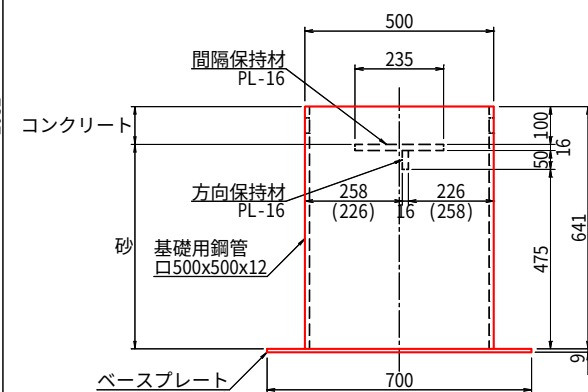
基礎用鋼管
