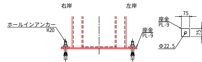
ホールインアンカー設置図
