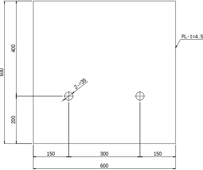
B1-5 調整プレート S=1/10
