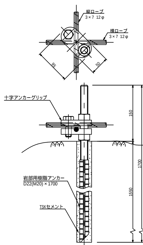
岩部用TSK樹脂アンカー
