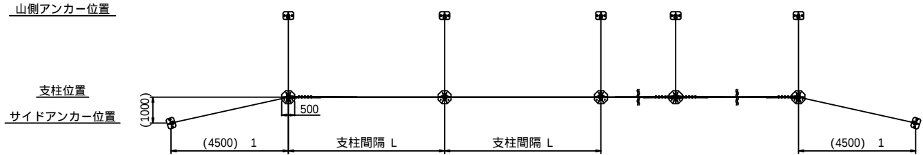
平面配置図 S=1/200
