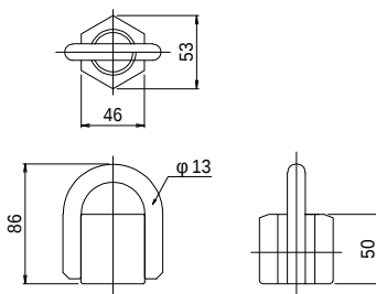
B4-2 フック付きナット
