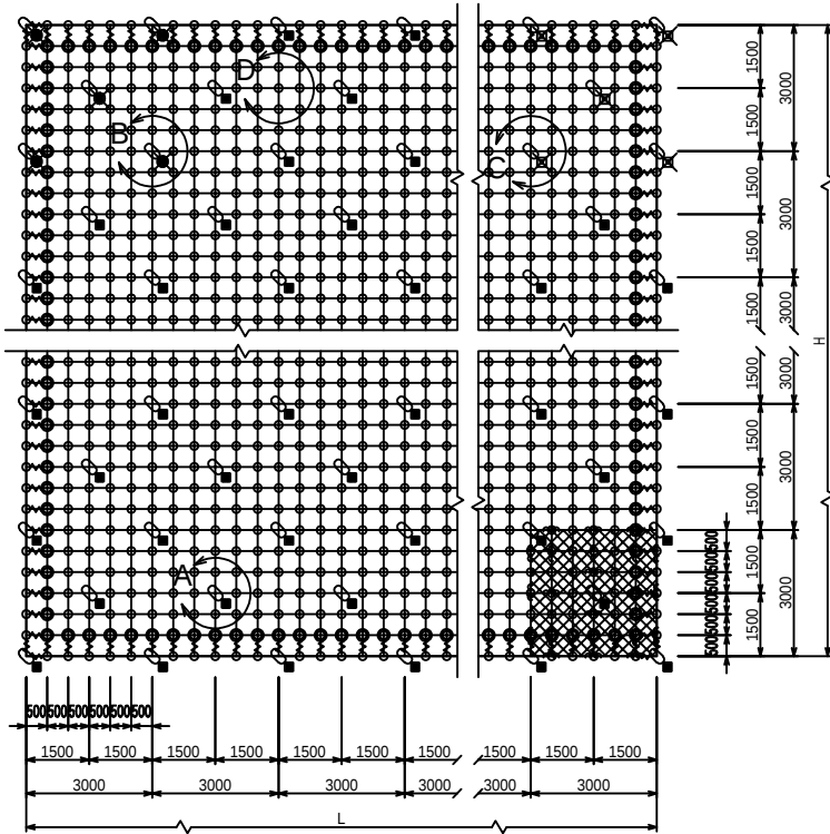
標準構造展開図
