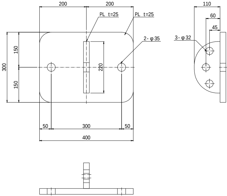
B1-6 アンカープレート S=1/10
