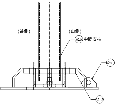
中間支柱・ベースプレートM組立図
