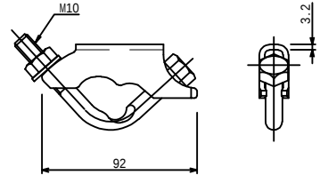
Vクリップ (大) (E部)
