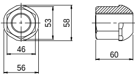
B1-2 ナット(球面) S=1/3 D29用
