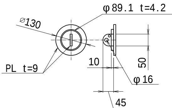
A1-2 支柱キャップ S=1/10
