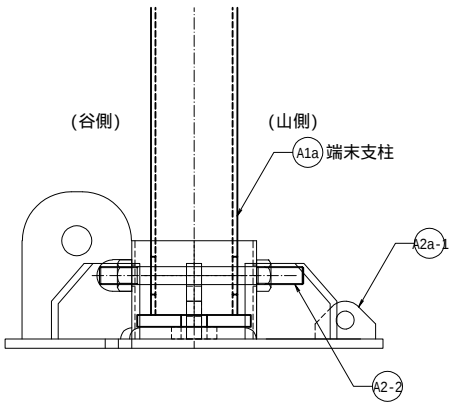
端末支柱・ベースプレートE組立図
