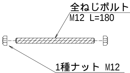
A1-3 全ねじボルト S=1/5 M12
