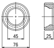
B1-3 ワッシャー(球面) S=1/3 D29用
