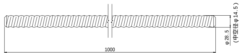
B4-1 自穿孔ロッド
