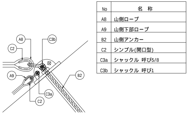
材料表(アンカー1組当たり)
