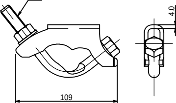
Vクリップ (大) (E部)
