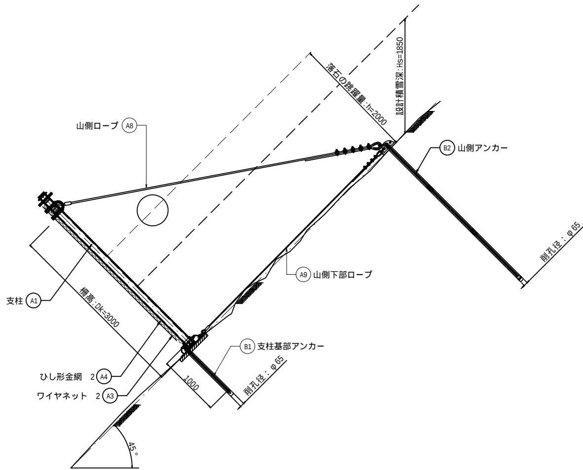
断面図 S=1/60
