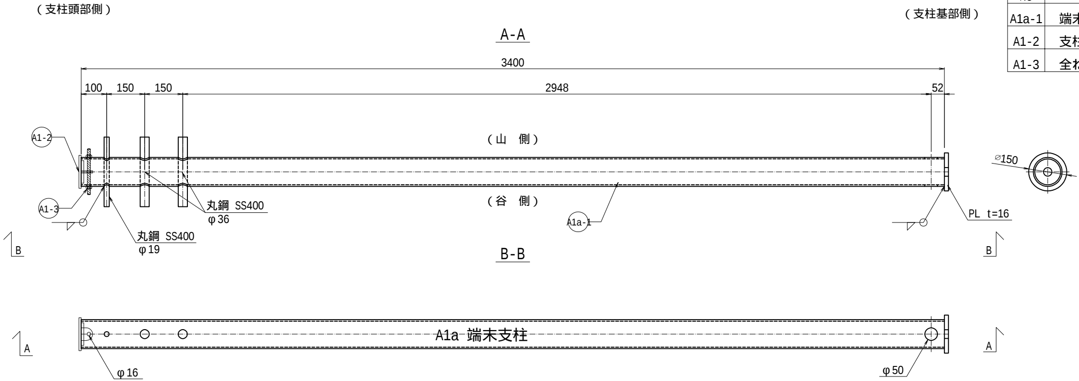
A1a 端末支柱 S=1/15
