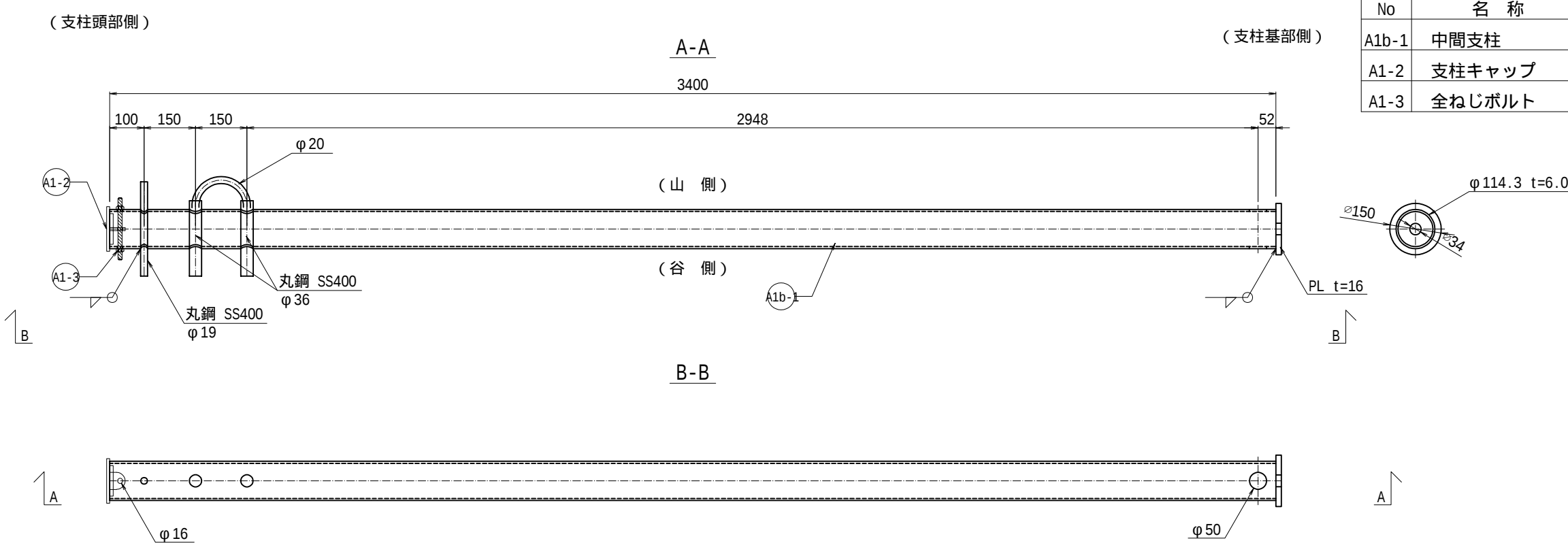
A1b 中間支柱 S=1/15
