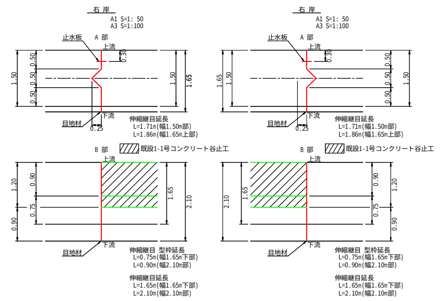
伸縮継目B 詳細図
