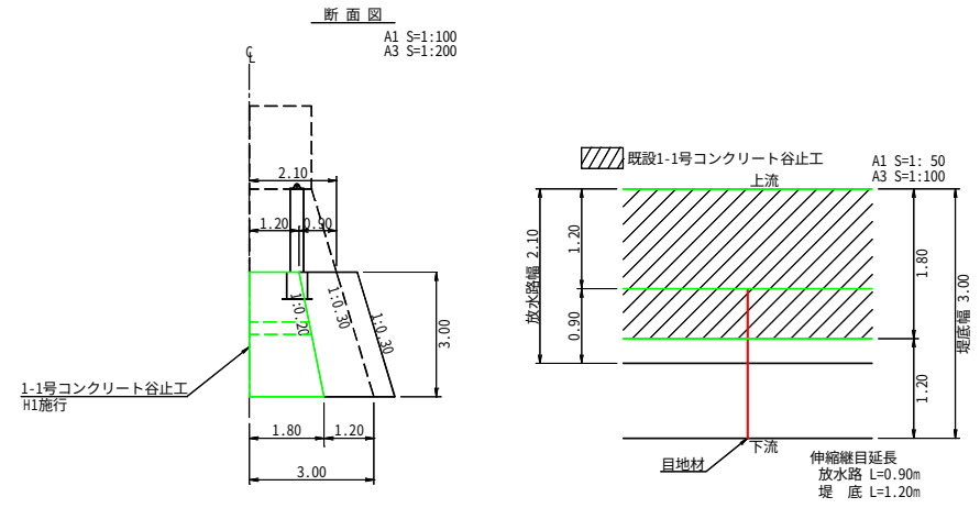
伸縮継目B 詳細図
