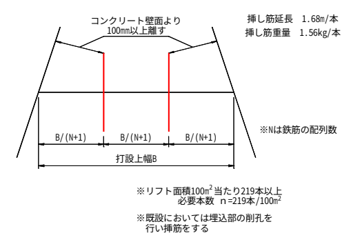
配置側面図
