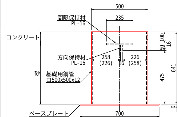
基礎用鋼管
