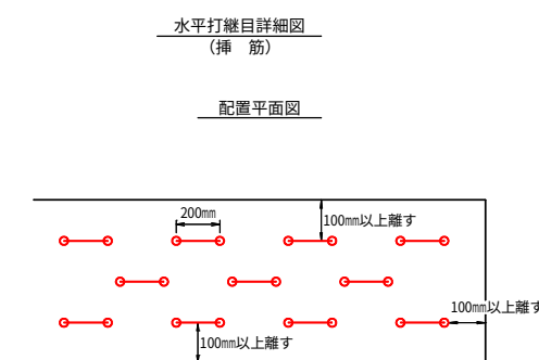
挿筋詳細図 D=16mm、SD295A
