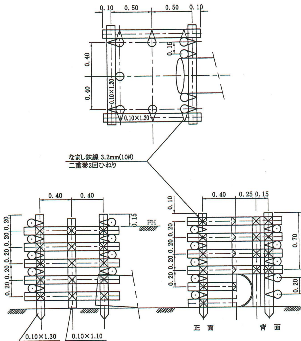
平 面 図
