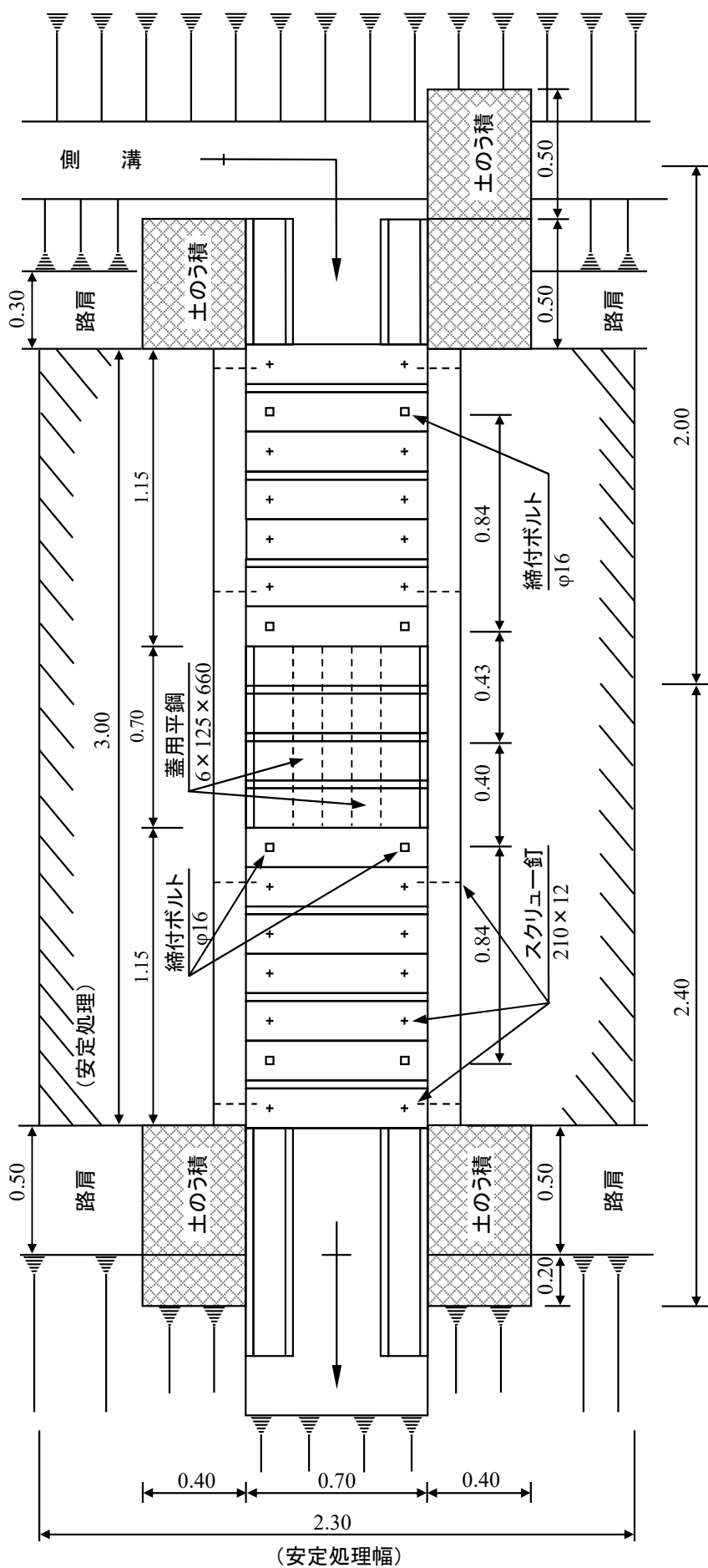
平 面 図
