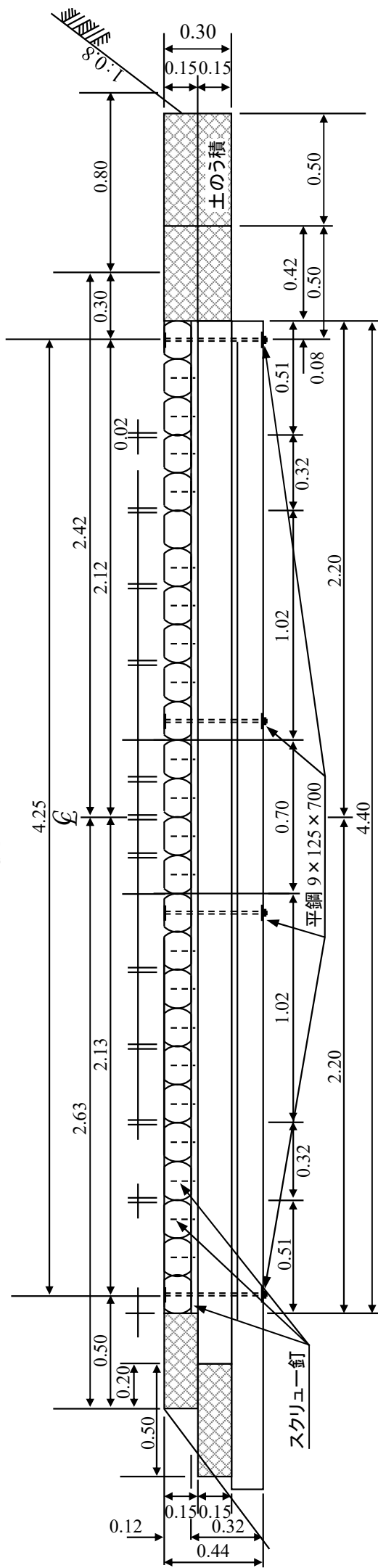
側面図
