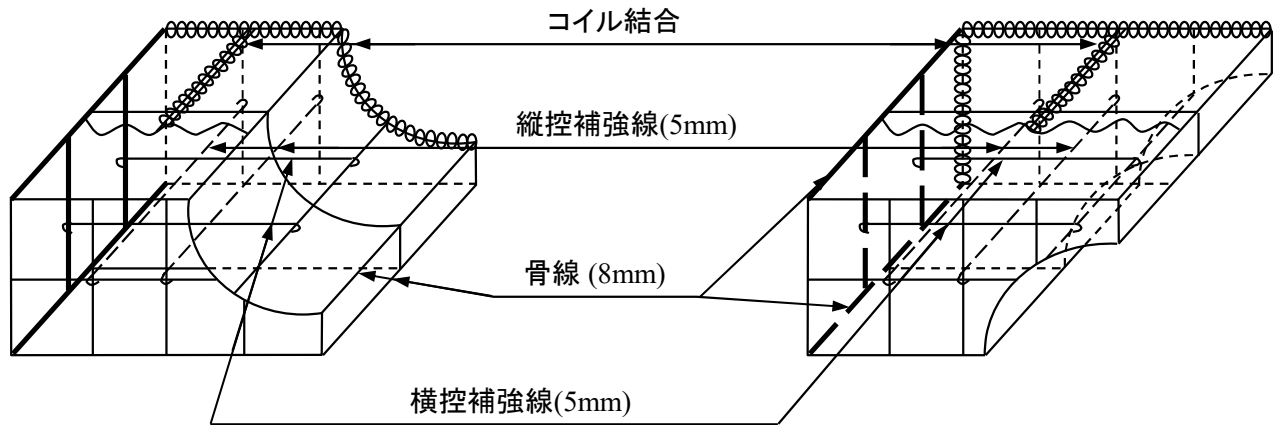
銅網パネル図(下部)
