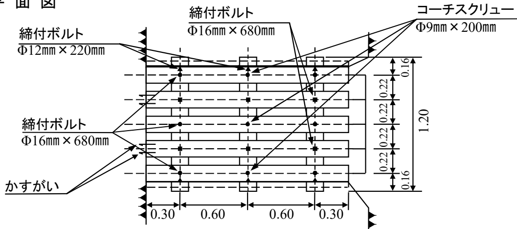
平面図
