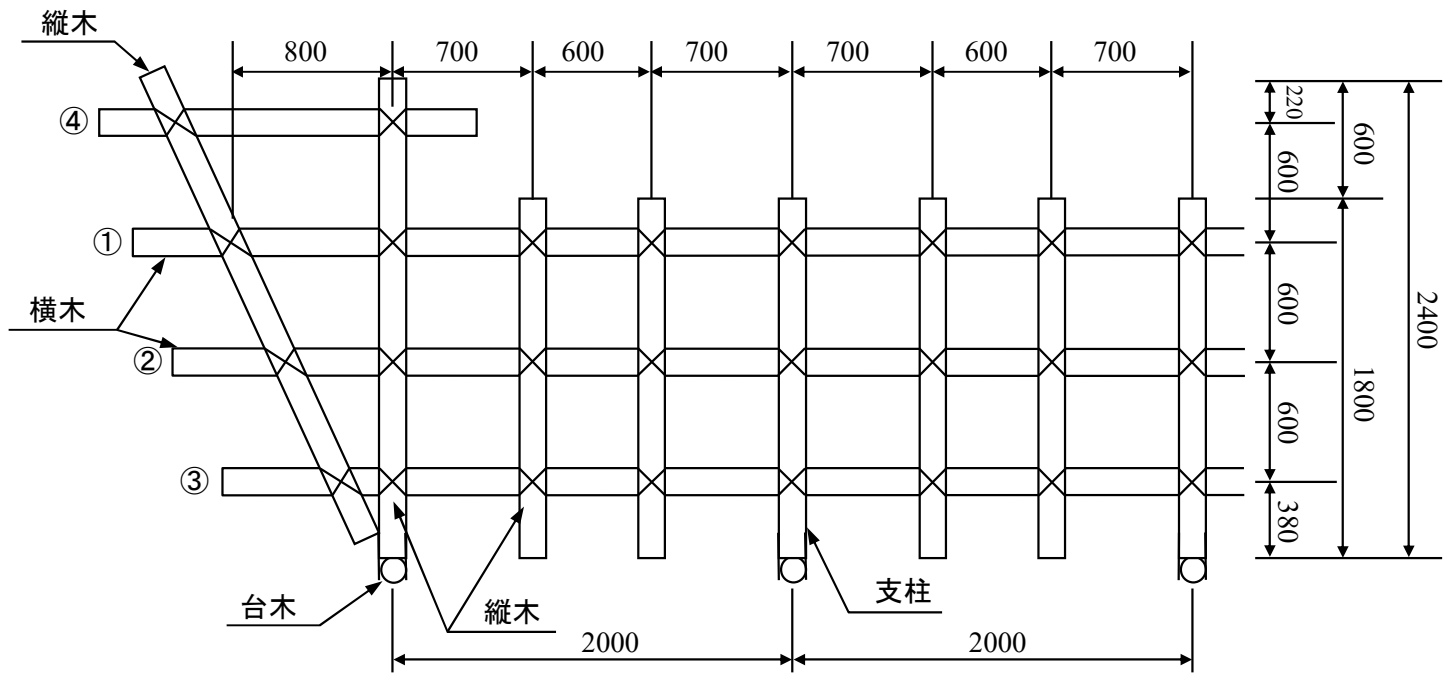
正面図
