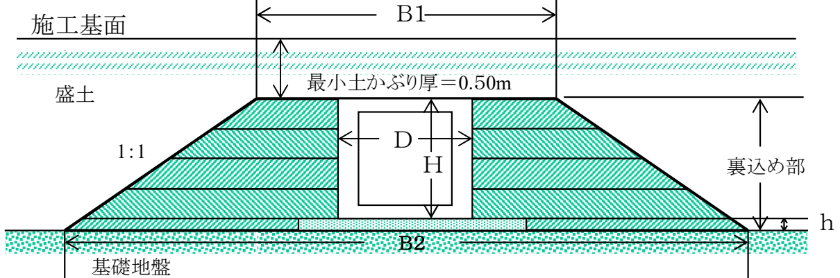
裏込め区域
