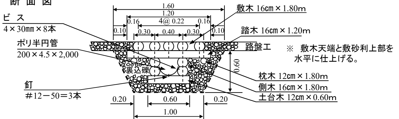
材料表
