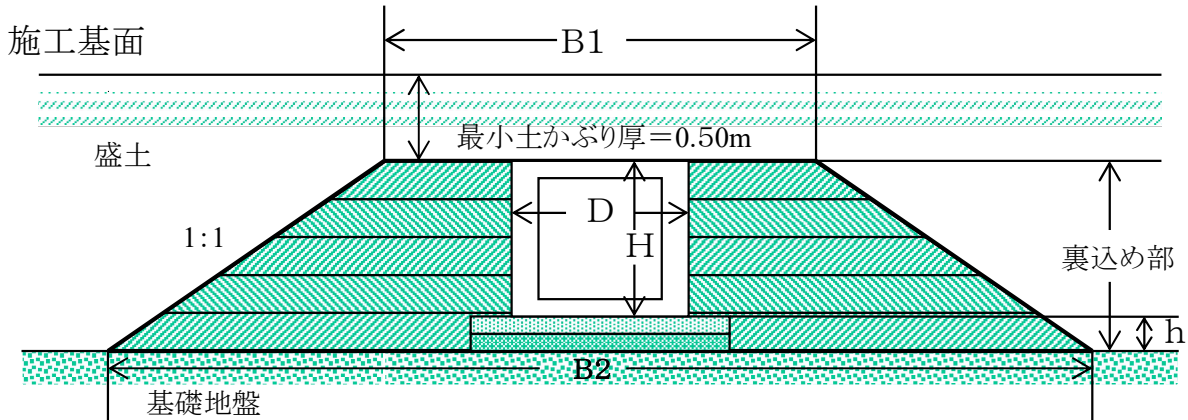
裏込め区域
