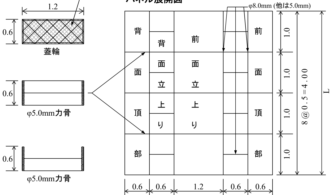
パネル展開図
