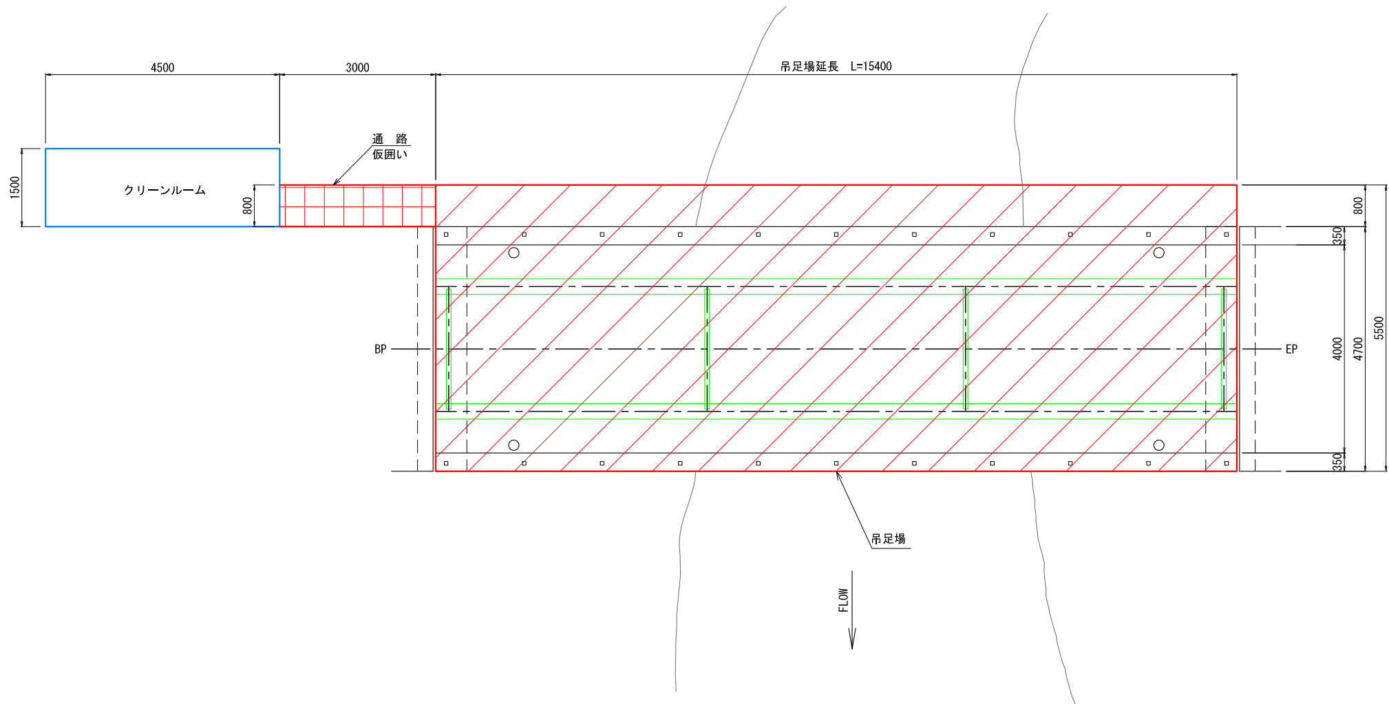
平面図 S=1:50
