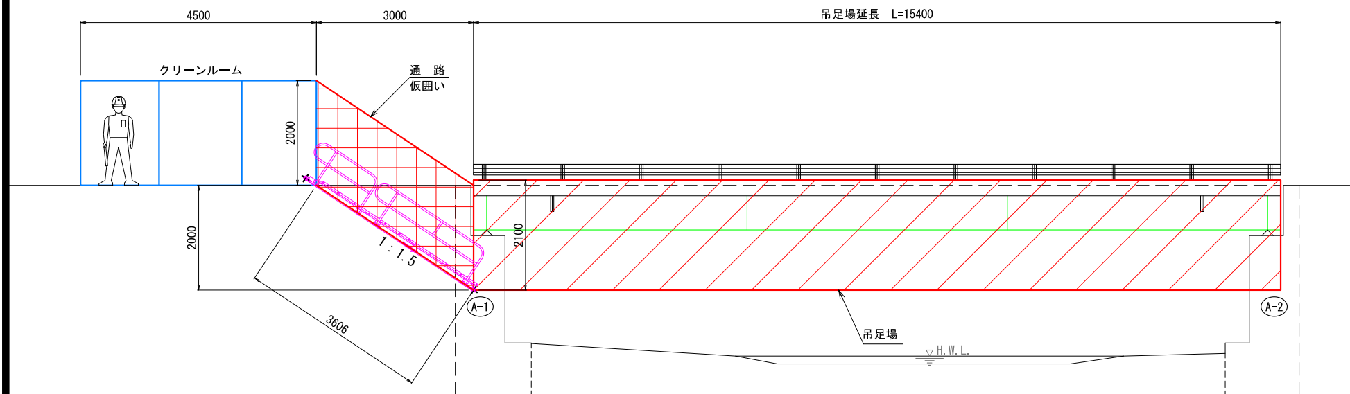
側面図 S=1:50
