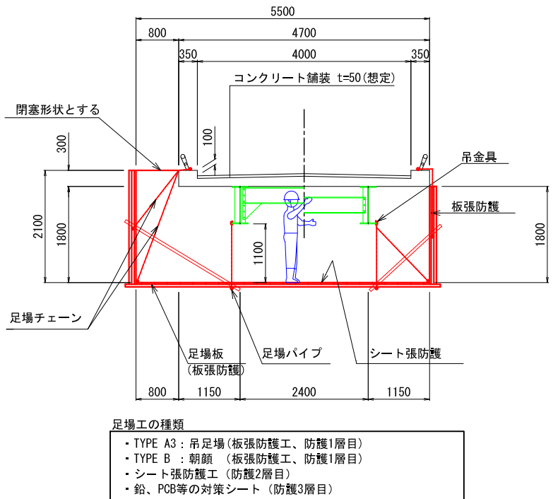
通路断面図 S=1:50
