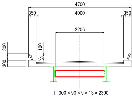
中間部 (2箇所)
