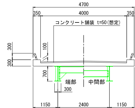
断面図 S=1:50
