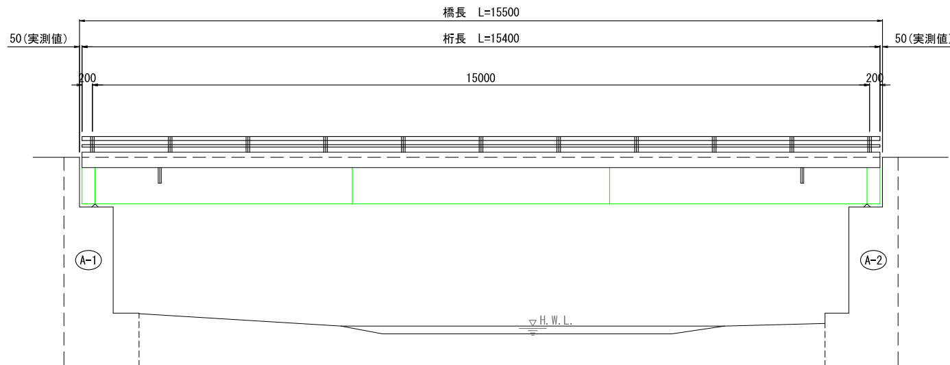
側面図 S=1:50
