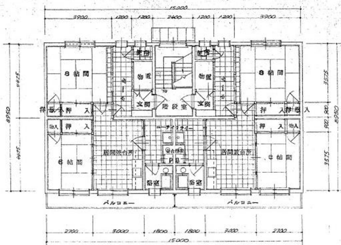
二階平面図
