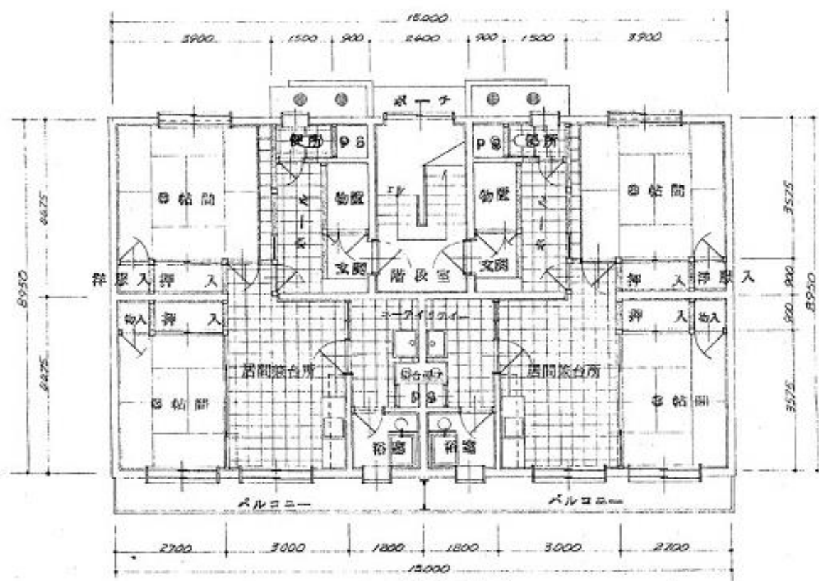
一階平面図
