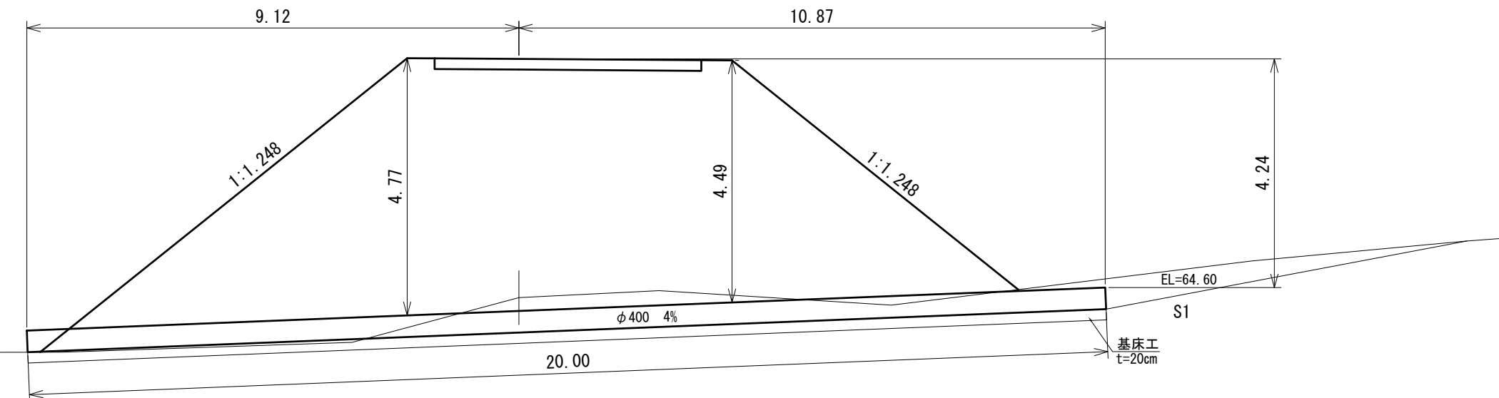
側面図
