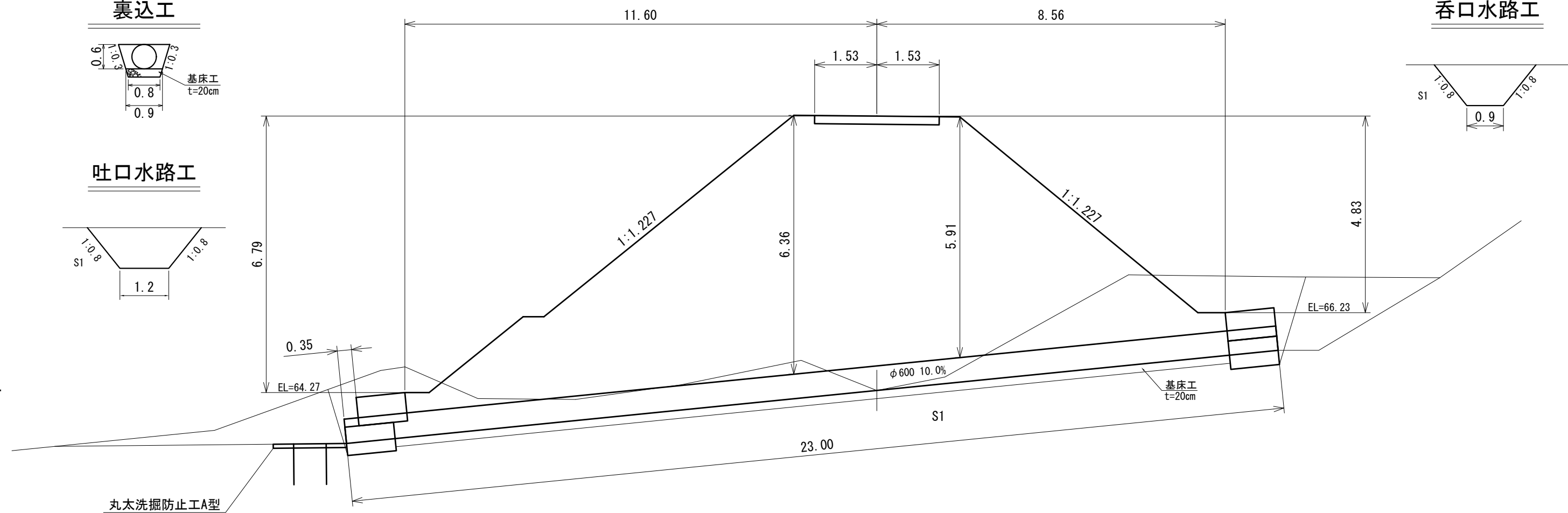
側面図
