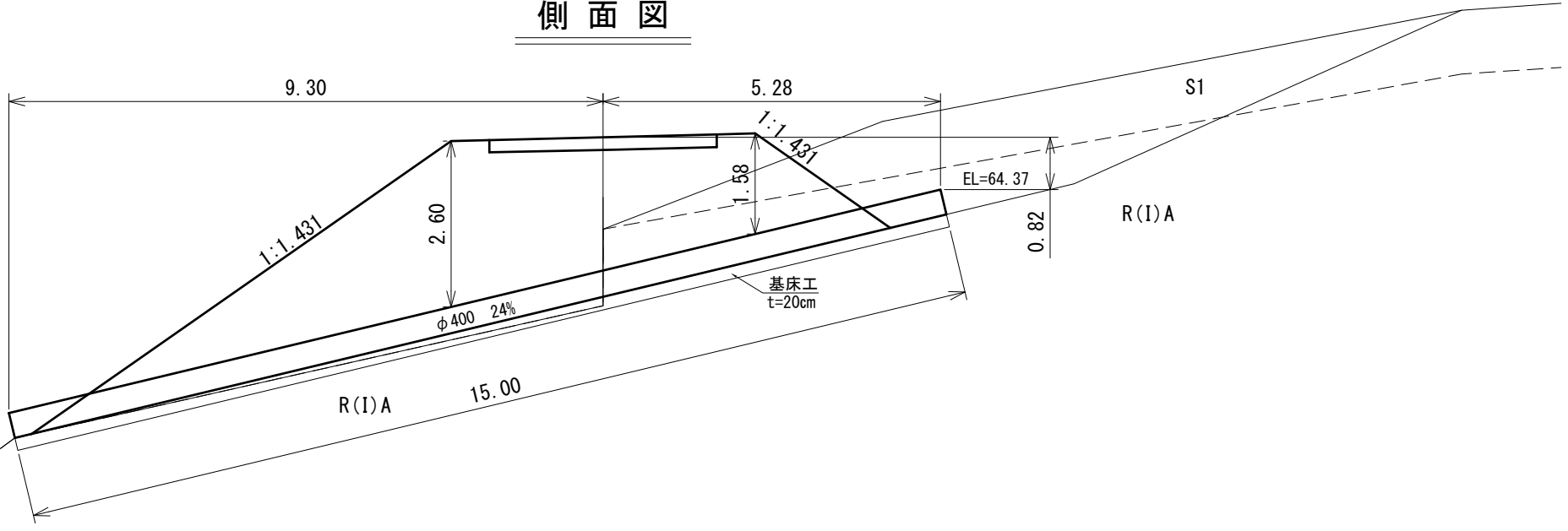
側面図
