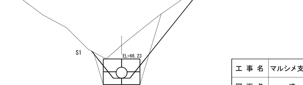
呑口正面図
