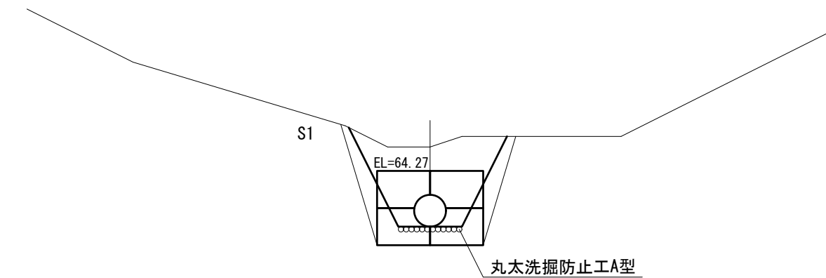
吐口正面図
