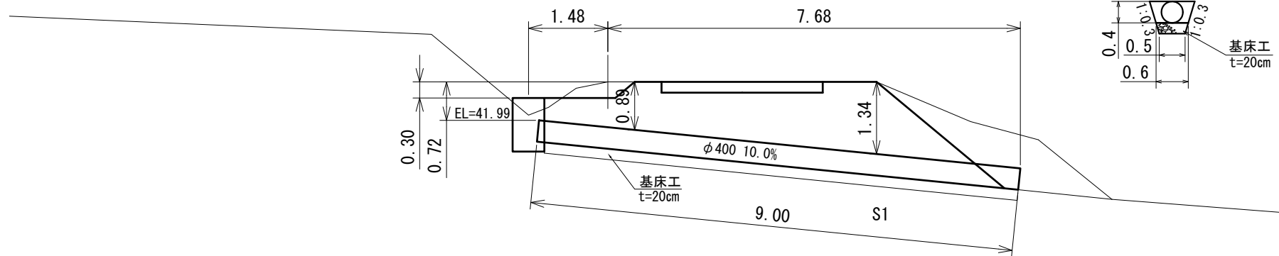
側面図
