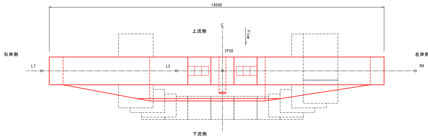
平面図
