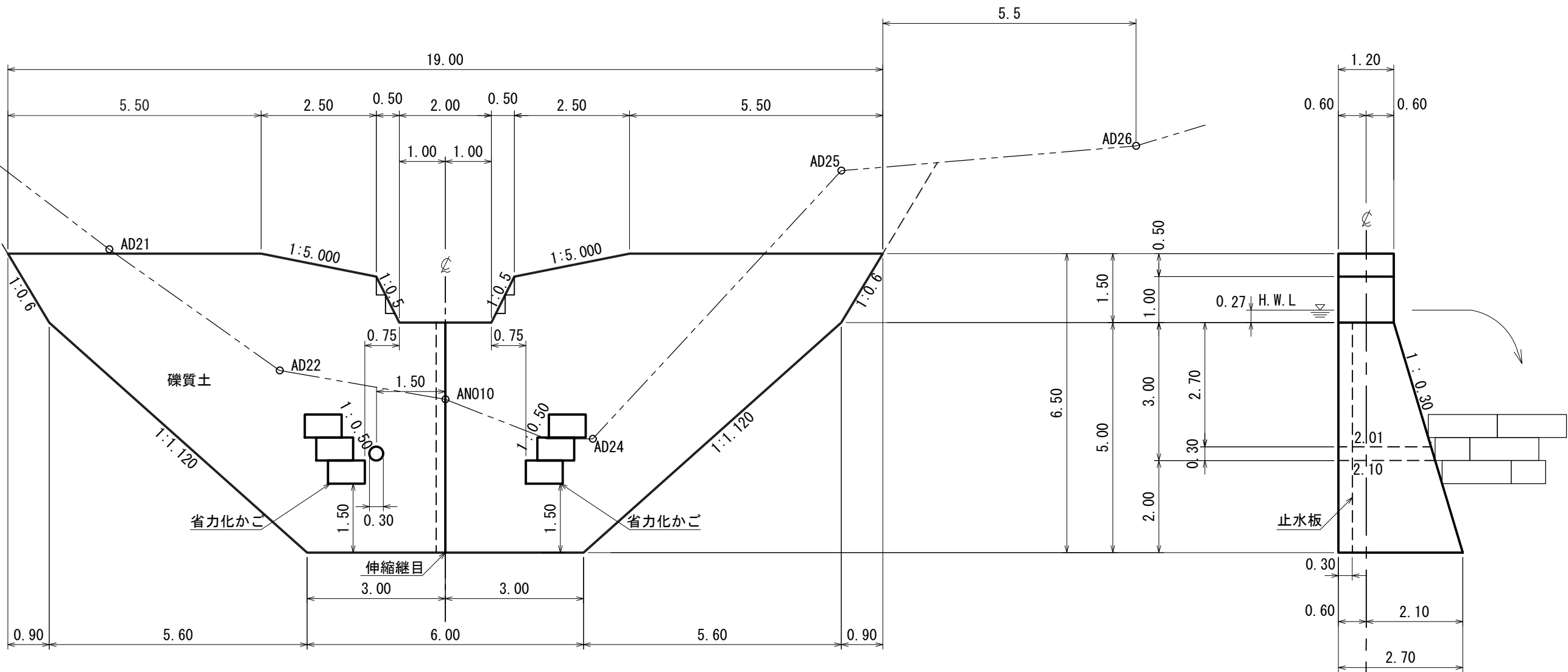
正面図
