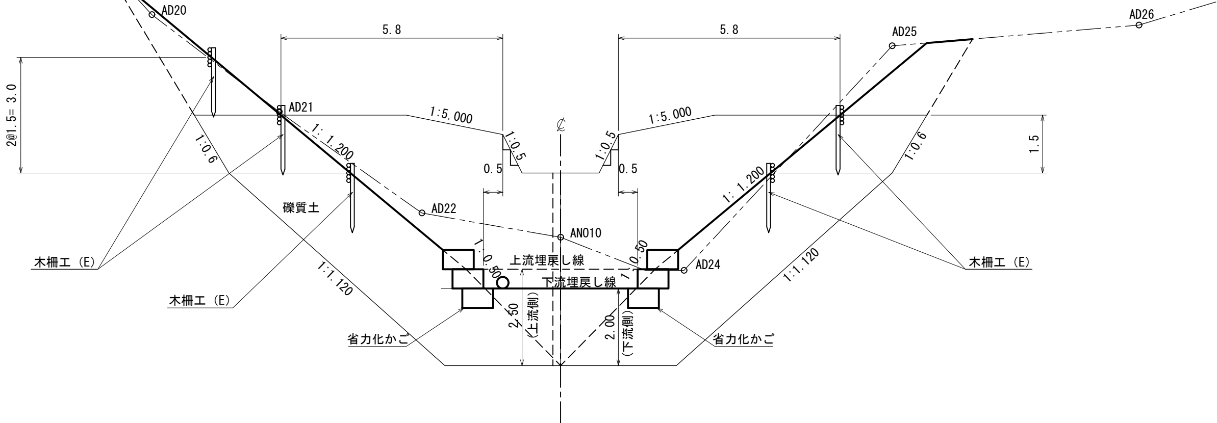
埋戻し図
