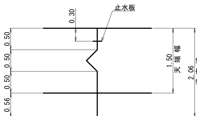
伸縮継目詳細図
