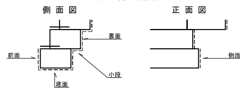
吸出し防止材設置図 (縮尺 任意)
