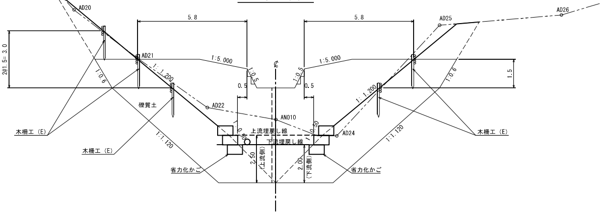
埋戻し図
