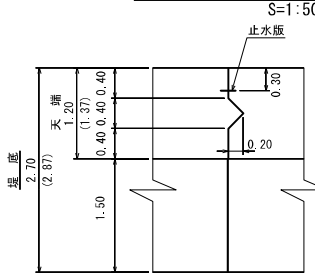
伸縮継目詳細図
