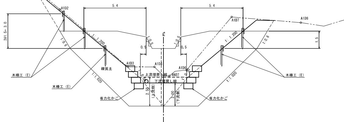
埋戻し図
