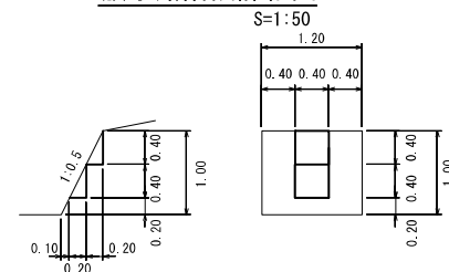
放水路階段詳細図
