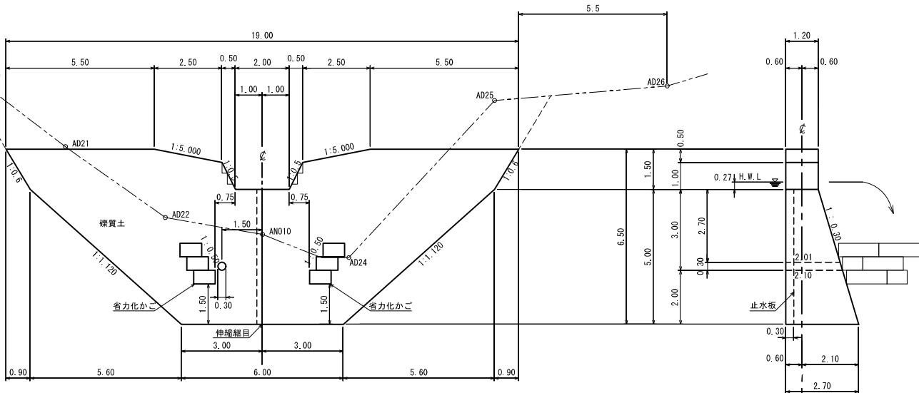
正面図
