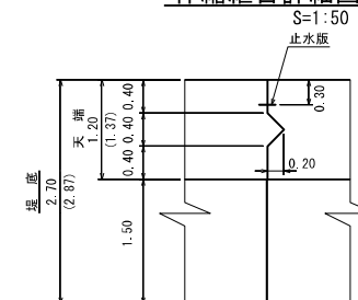
伸縮継目詳細図
