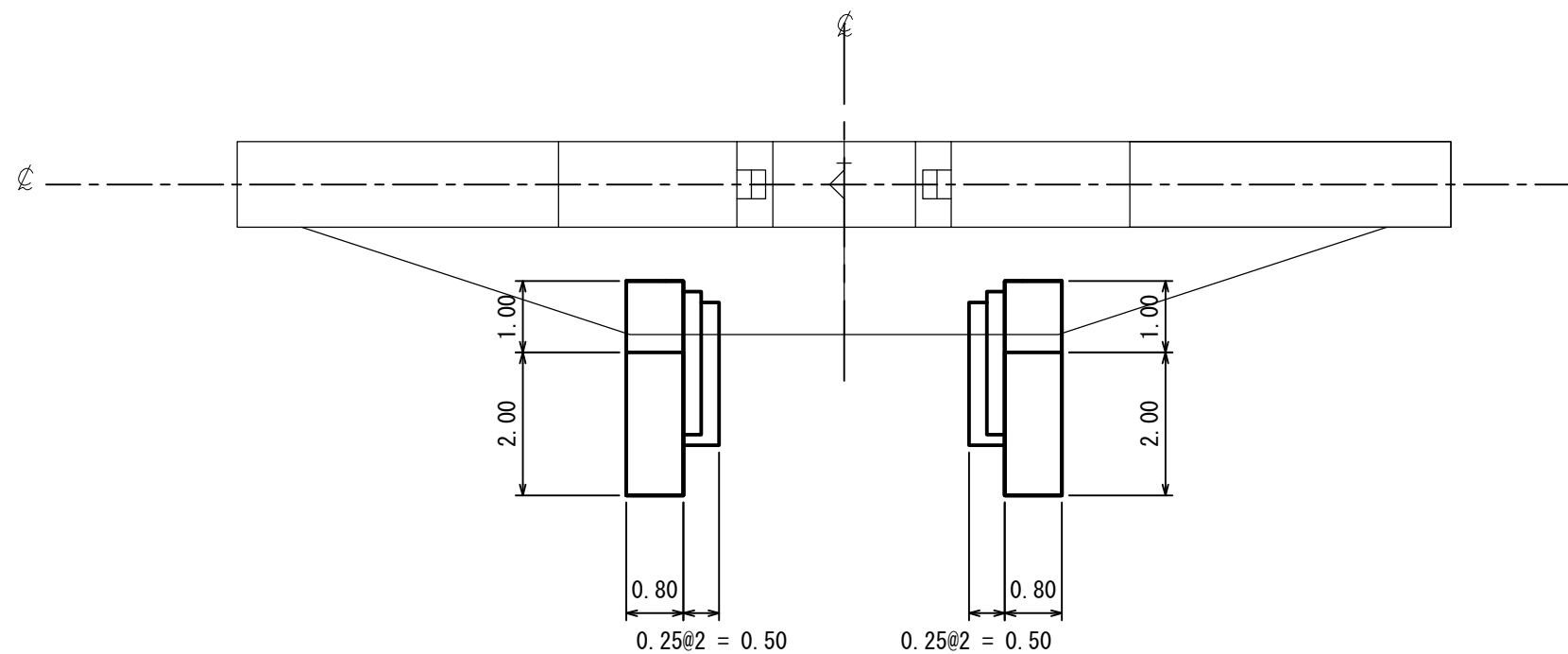
平面図
