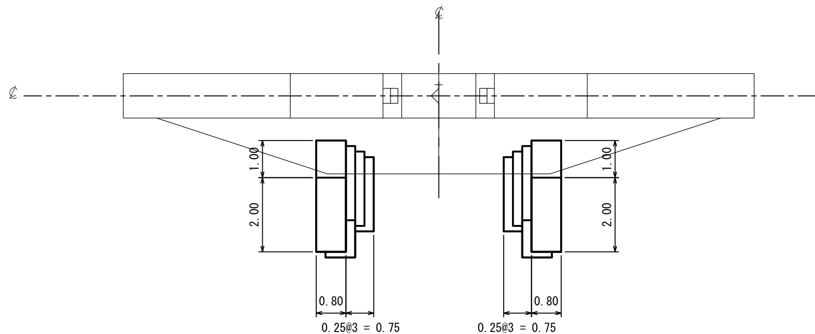
平面図
