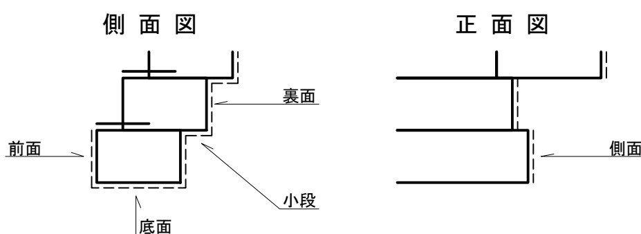
吸出し防止材設置図 (縮尺 任意)
