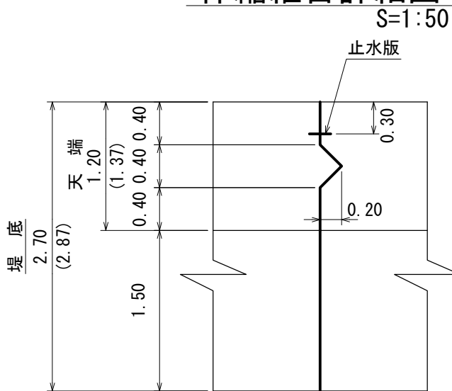
伸縮継目詳細図
