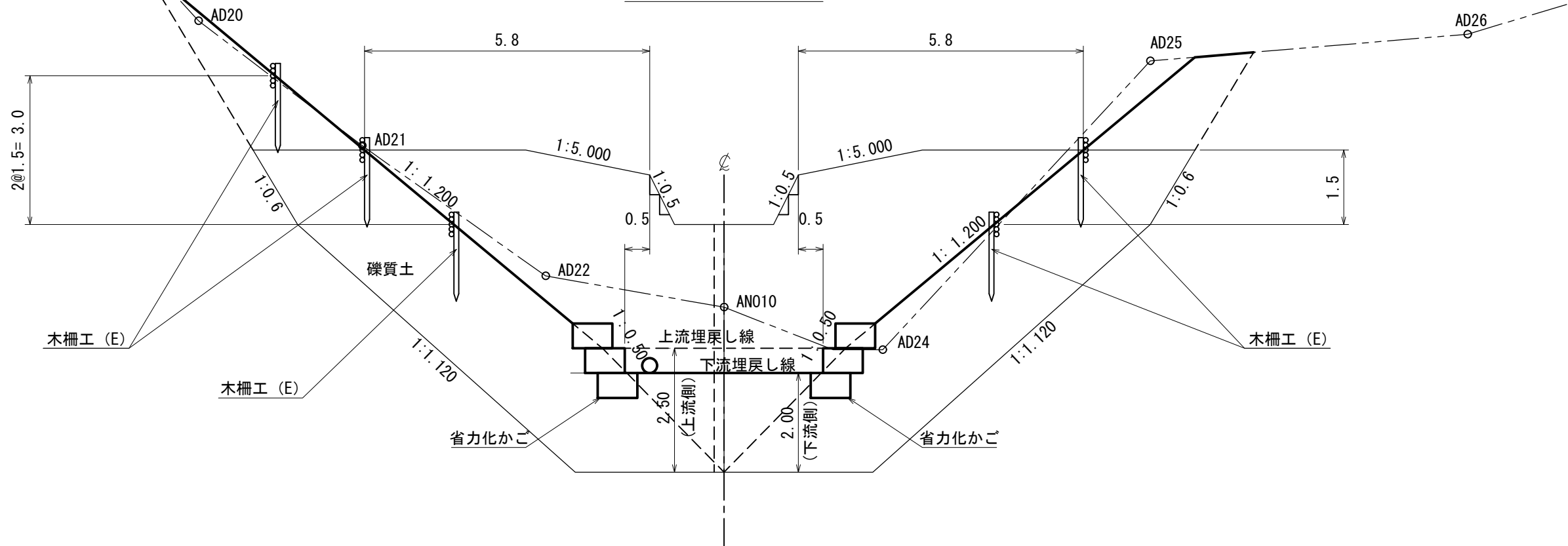
埋戻し図
