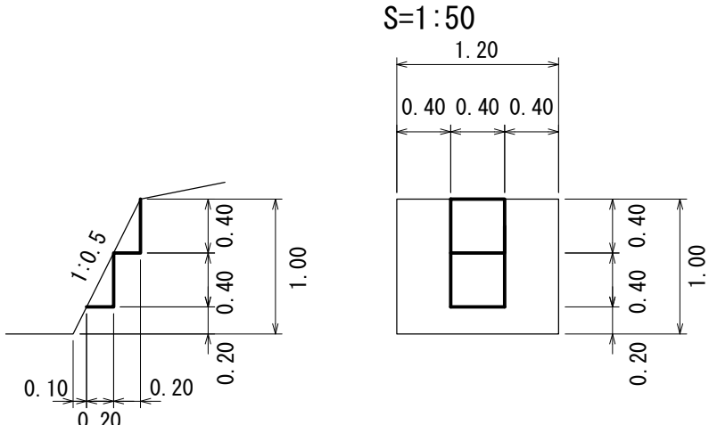
放水路階段詳細図
