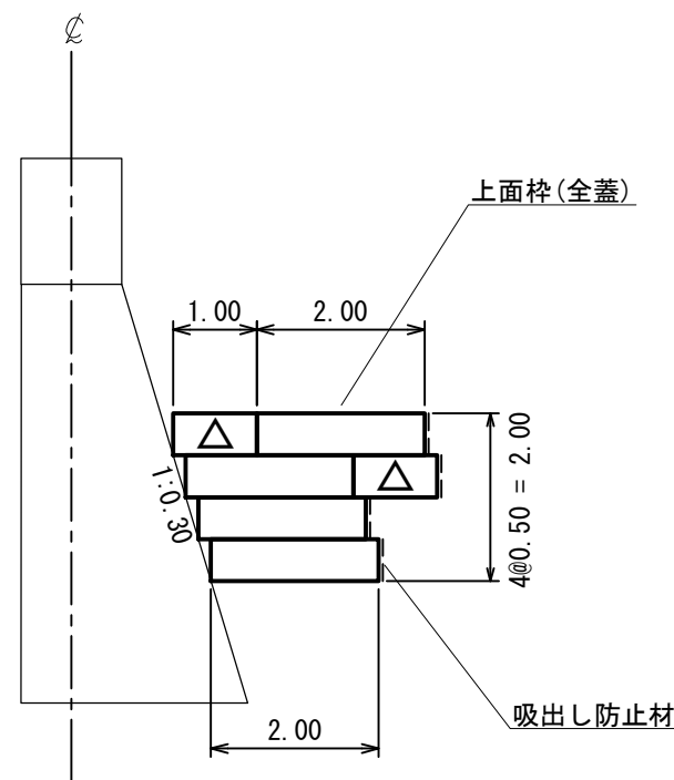
正面図
