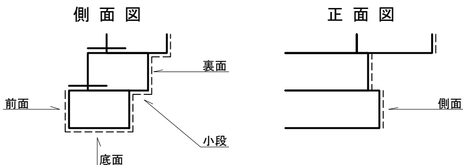
吸出し防止材設置図 (縮尺 任意)
