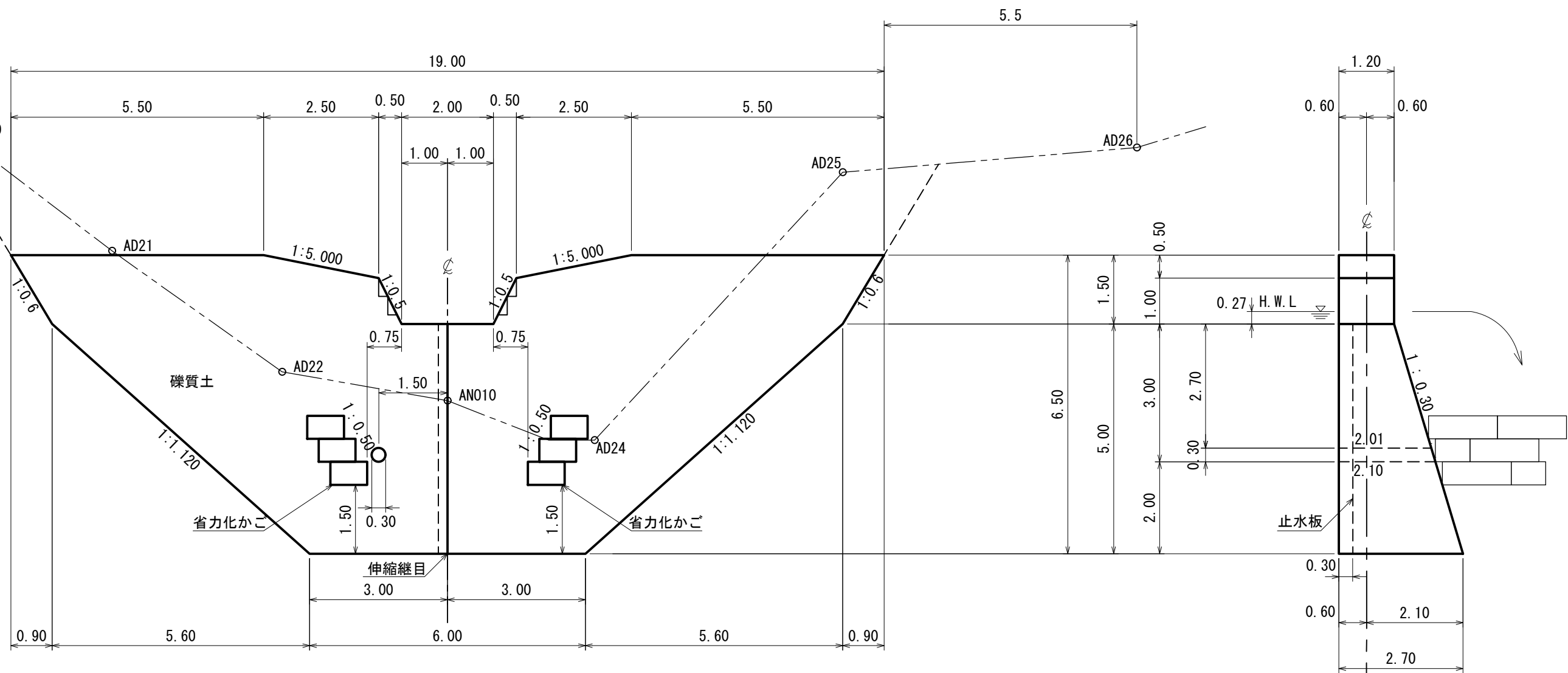
正面図
