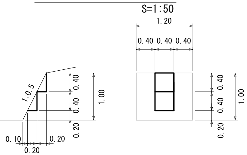
放水路階段詳細図
