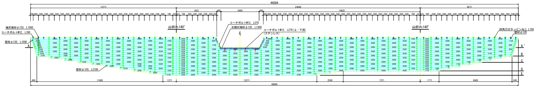
正面図 (b-b)
