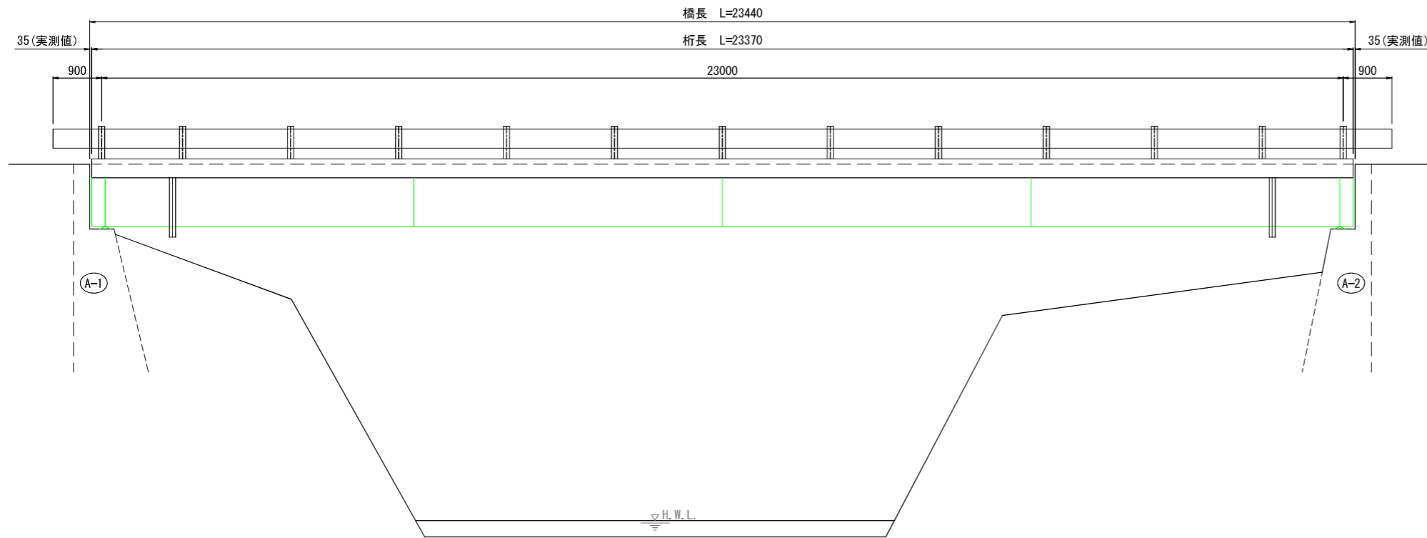
側面図 S=1:50
