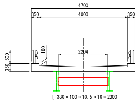
中間部 (3箇所)
