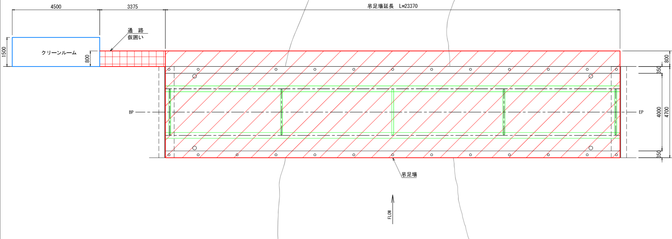
平面図 S=1:60
