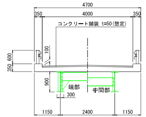
断面図 S=1:50
