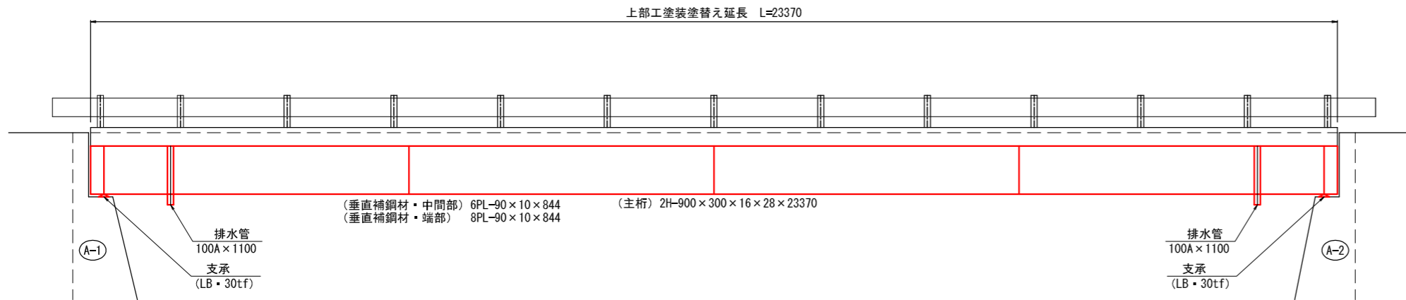
断面図 S=1:50
