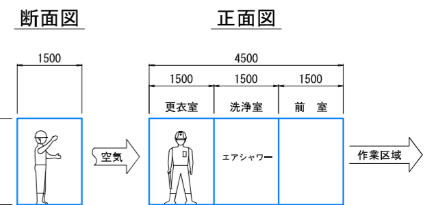
クリーンルーム模式図(案) S=1:60
