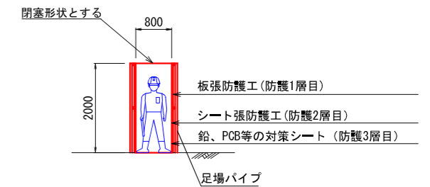
クリーンルーム模式図(案) S=1:60
