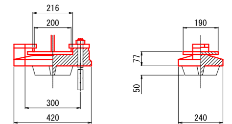
線支承 (LB・30tf) 可動 (2箇所) S=1:10
