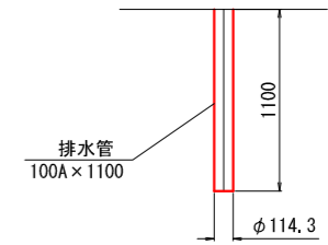
排水管 (4箇所) S=1:25
