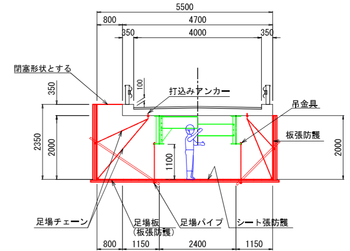
吊足場断面図 S=1:60
