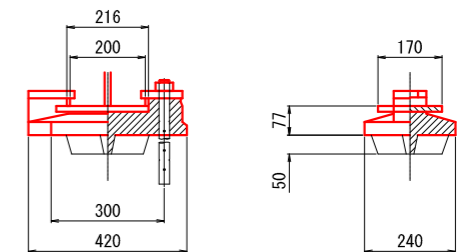
線支承 (LB・30tf) 固定 (2箇所) S=1:10
