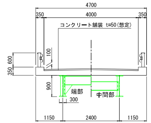
断面図 S=1:50
