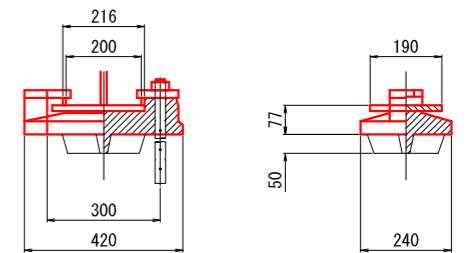
線支承 (LB・30tf) 可動 (2箇所) S=1:10
