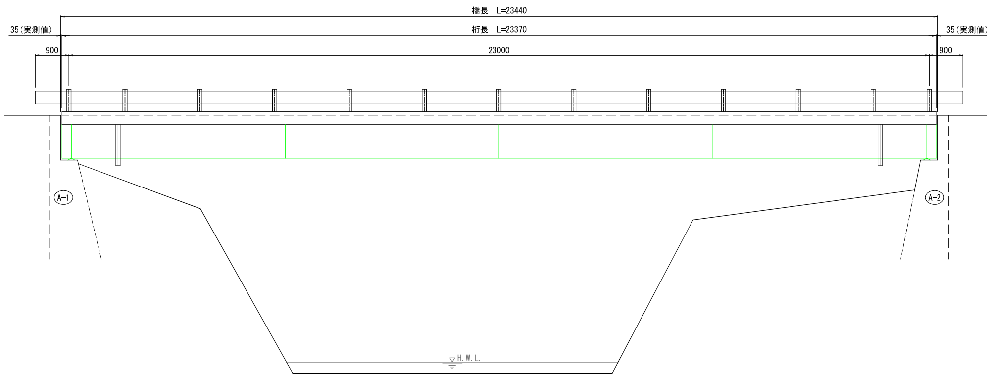
側面図 S=1:50
