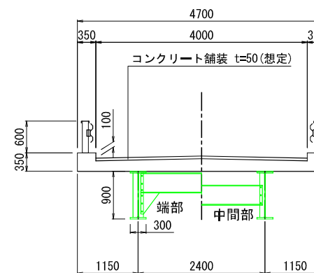
断面図 S=1:50
