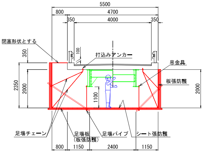
吊足場断面図 S=1:60
