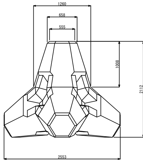
●正面図
