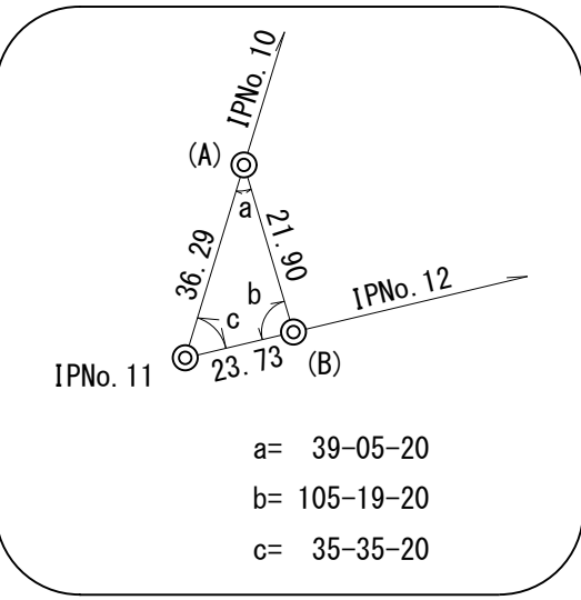
IPNO . 11詳細図
