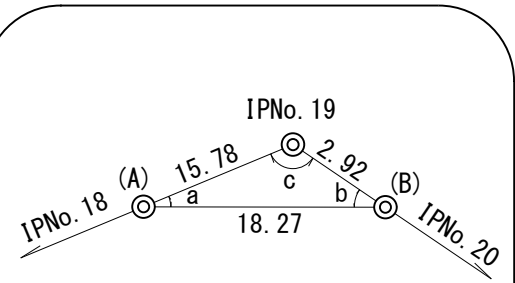
IPNO . 19詳細図
