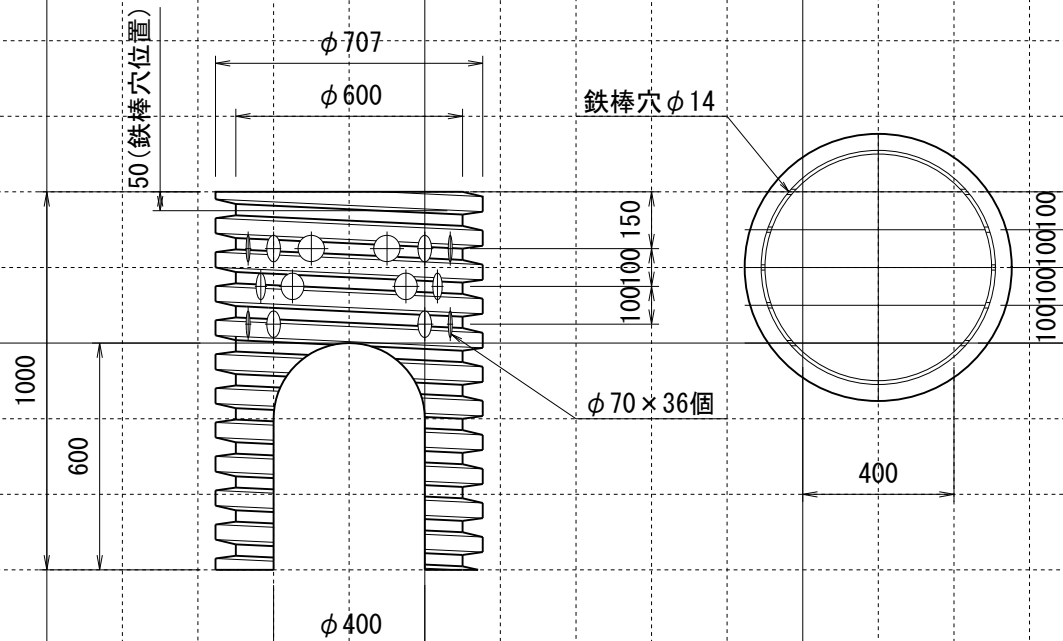
ポリ集水桝標準図 φ400用
