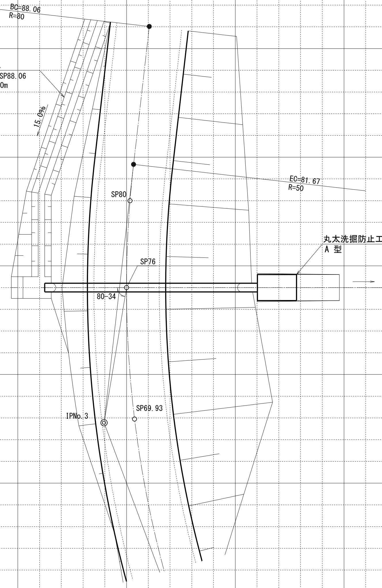
側溝工
