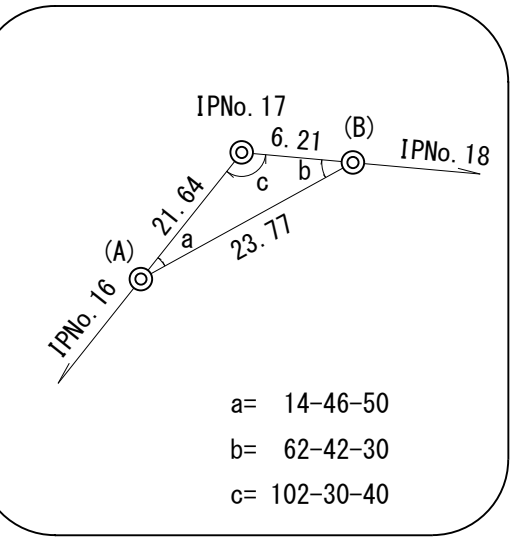
IPNO . 17詳細図
