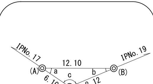
IPNO . 18詳細図
