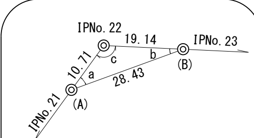
IPNO . 22詳細図
