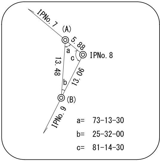
IPNO . 8詳細図
