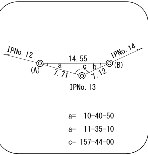
IPNO . 13詳細図
