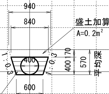
管基礎標準図 半溝型
