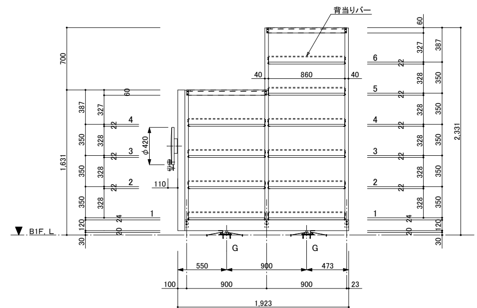
移動棚 側面図 【有効4段/6段】 S = 1 ; 30
