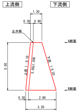
伸縮継目1 断面図
