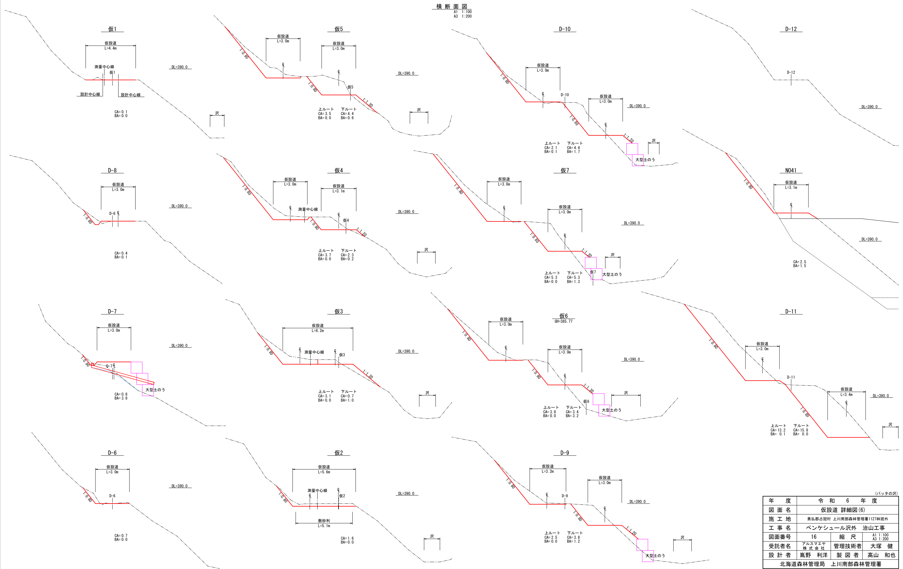
仮設道 詳細図(6)
