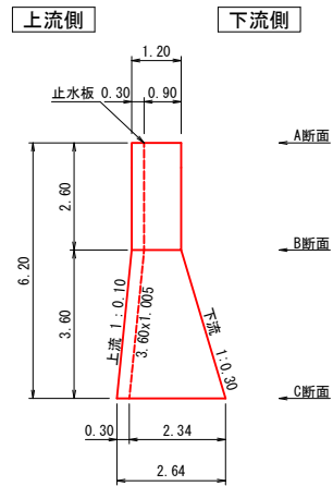
伸縮継目3 断面図
