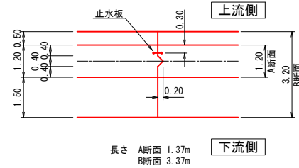
伸縮継目1平面図
