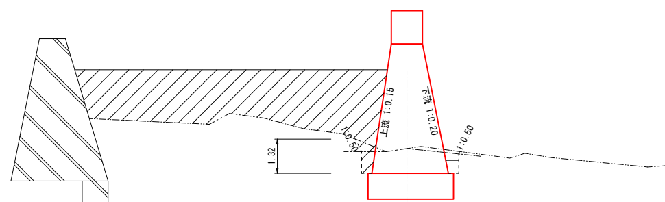
第1号コンクリート堰堤工 (S38)
