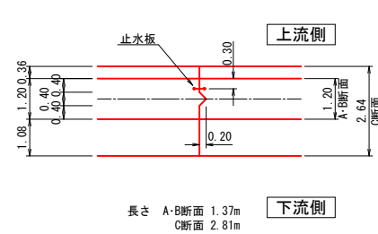
伸縮継目3平面図
