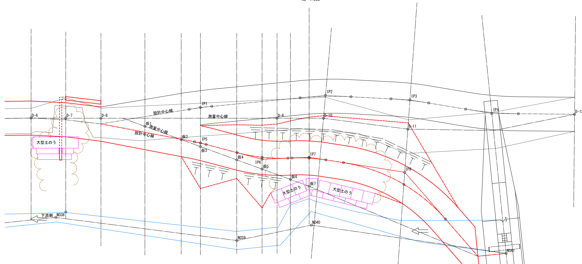
縦断面図 A1 1:100 A3 1:200
