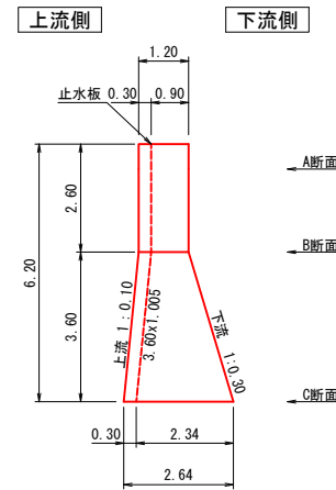
伸縮継目4 断面図
