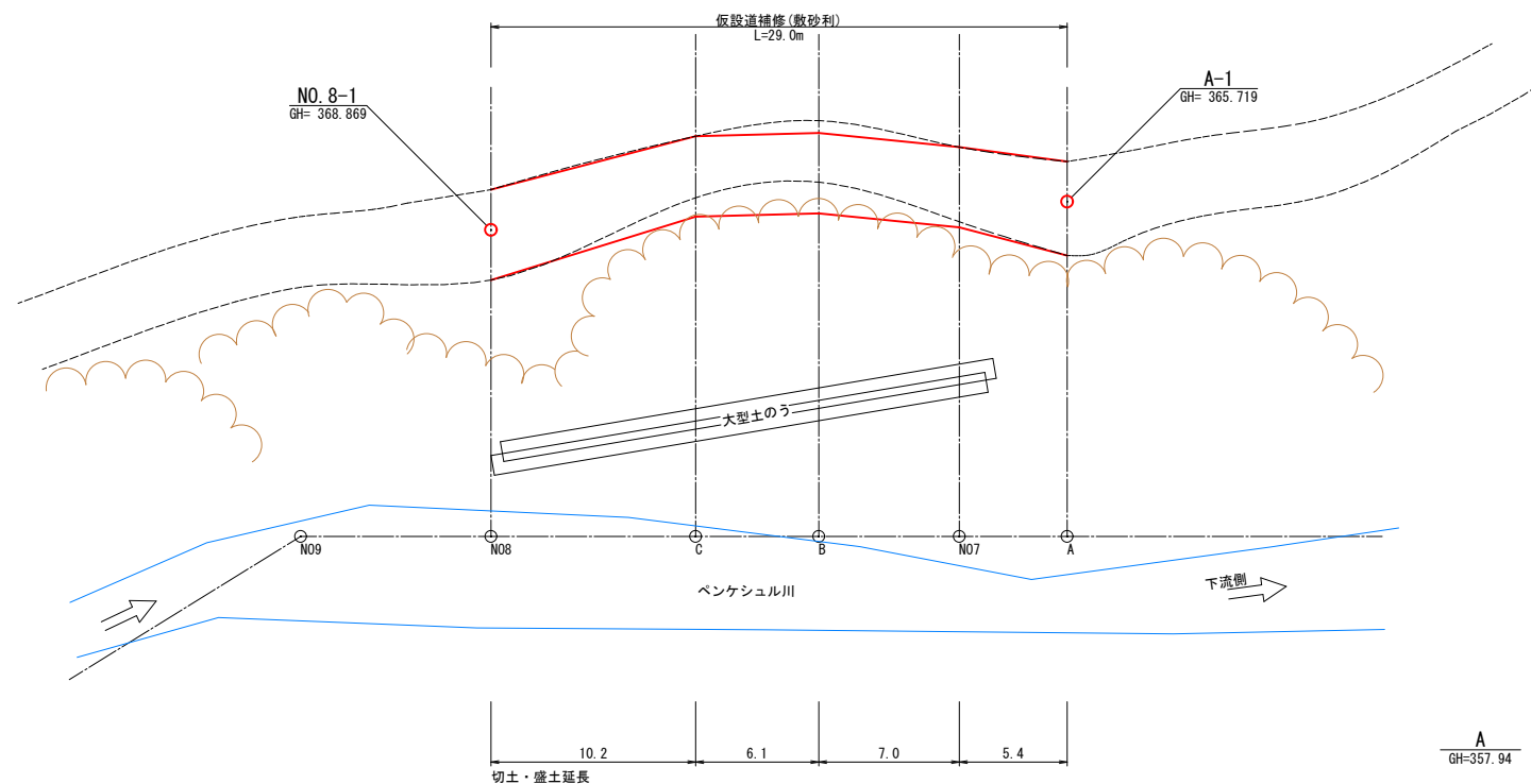
平面図 A1 1:200 A3 1:400
