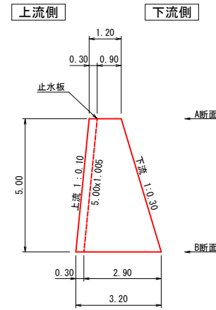
伸縮継目2 断面図
