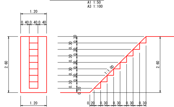
放水路階段詳細図
