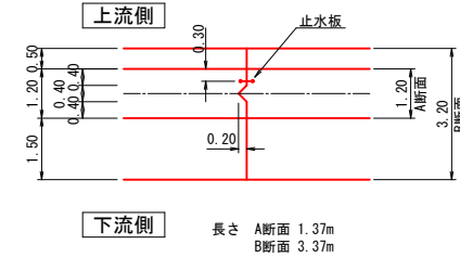
伸縮継目2平面図
