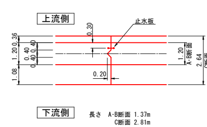
伸縮継目4平面図
