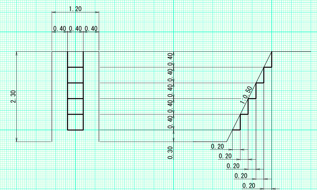
放水路階段詳細図
