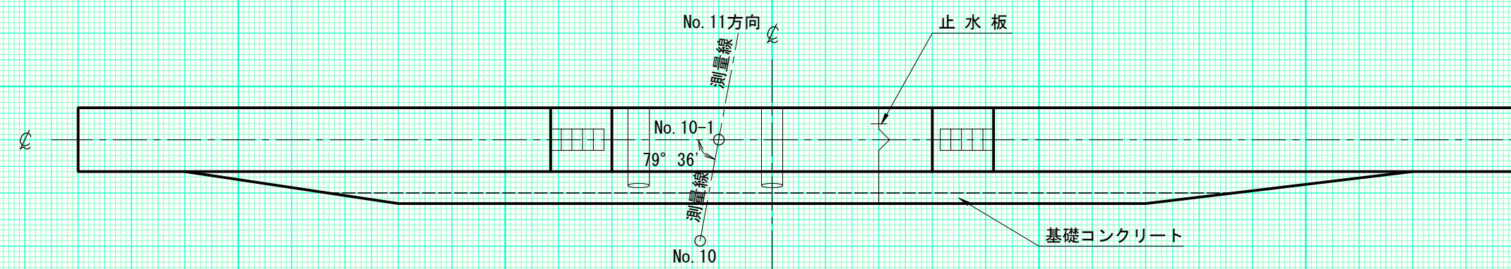
平面图
