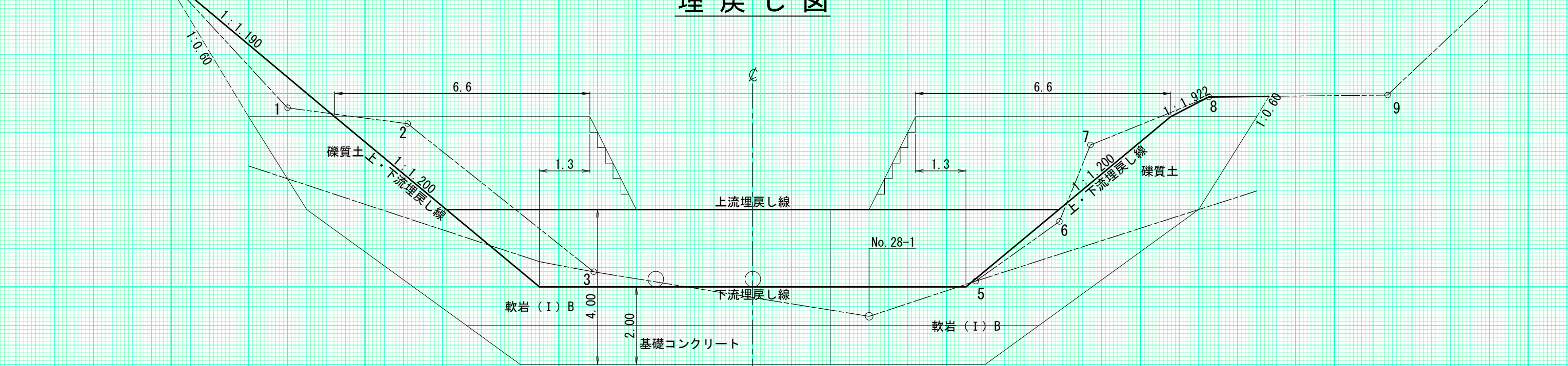
埋戻し図
