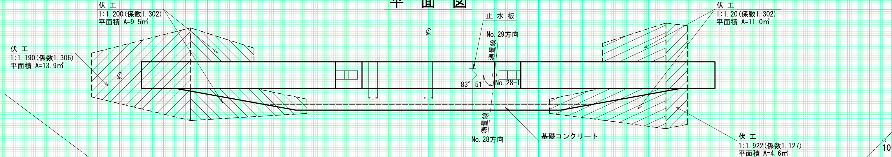
埋戻し図
