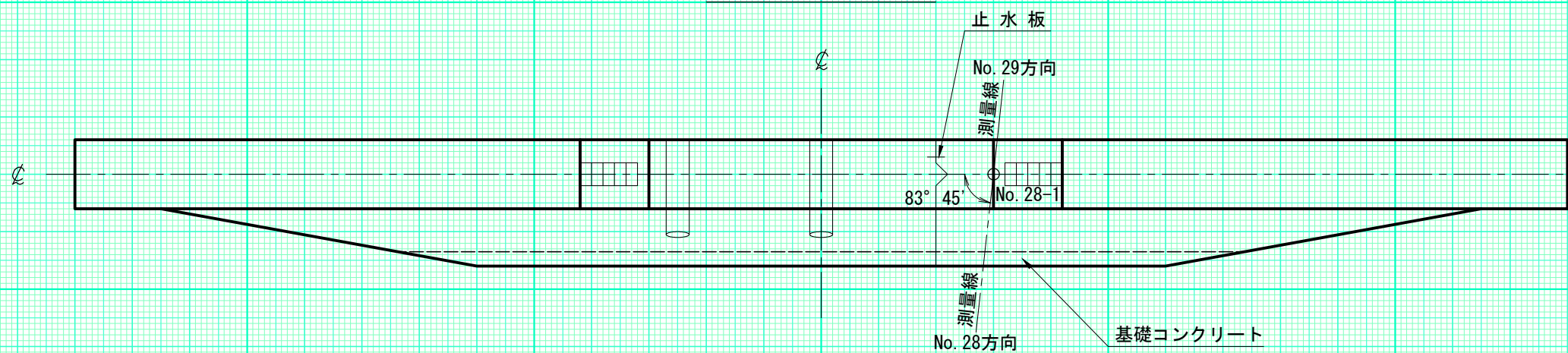
平面図
