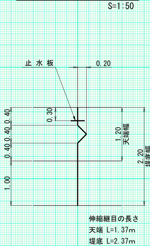
伸縮継目詳細図
