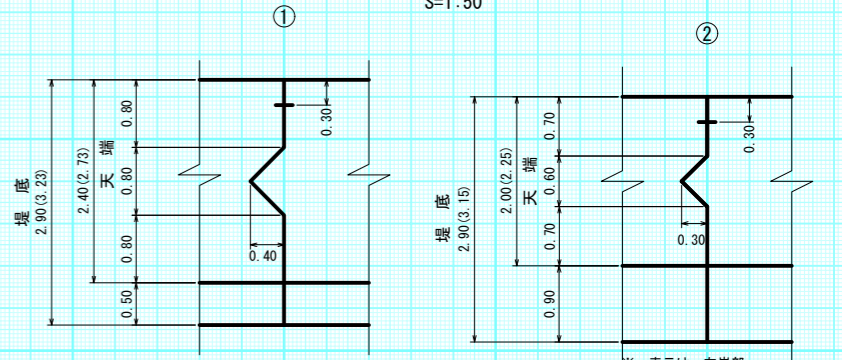
伸縮継目詳細図 S=1:50
