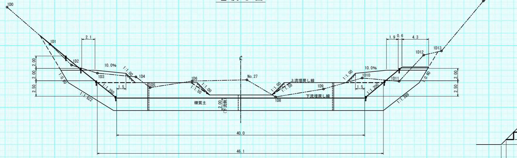
埋戻し図
