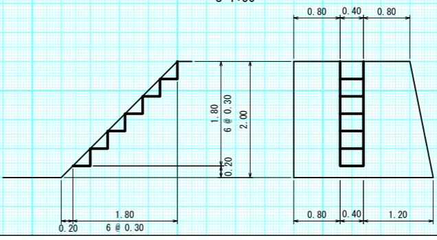
複断面放水路階段詳細図 S=1:50
