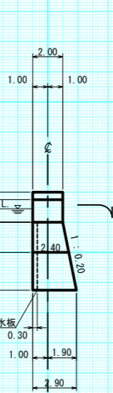
側面図
