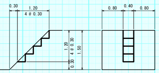
放水路階段詳細図 S=1:50
