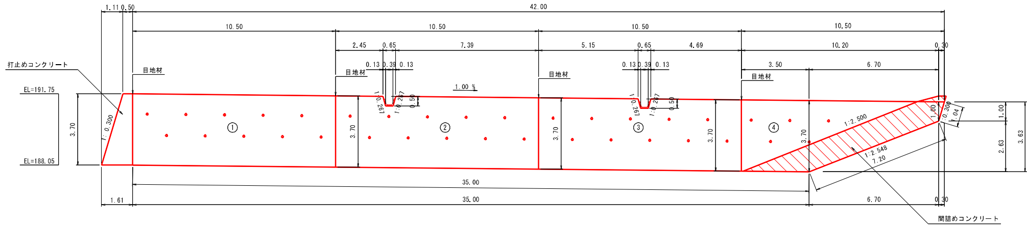
正面図
