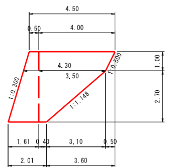
側 面 図
