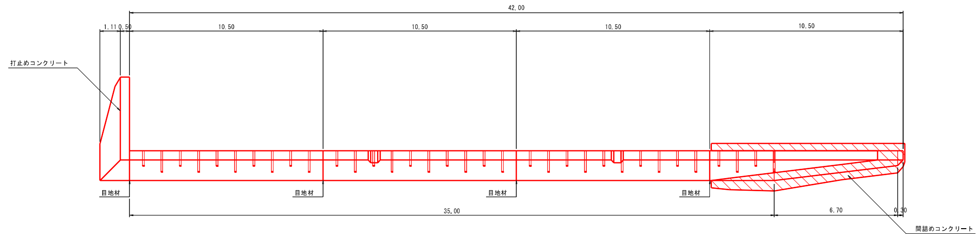
平面图
