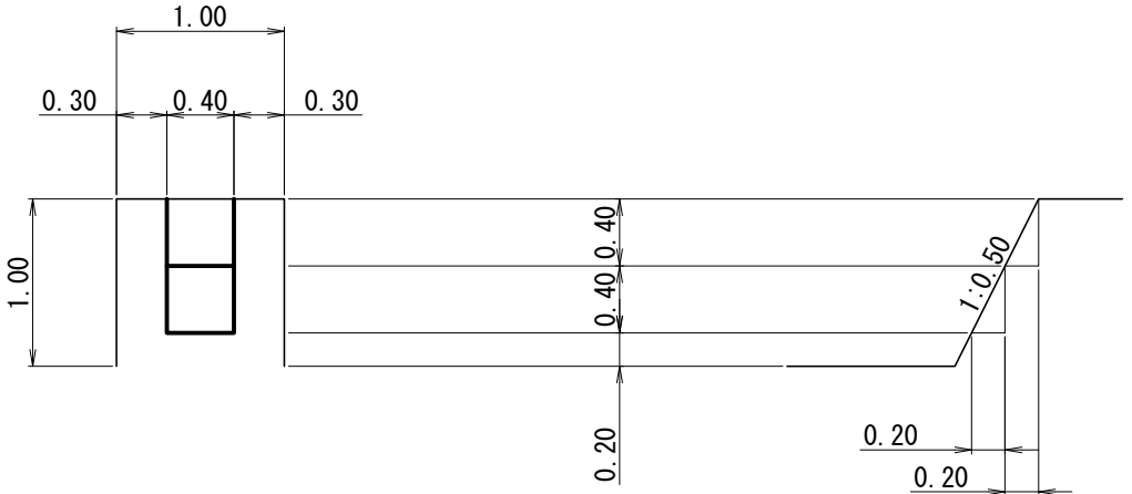
放水路階段詳細図
