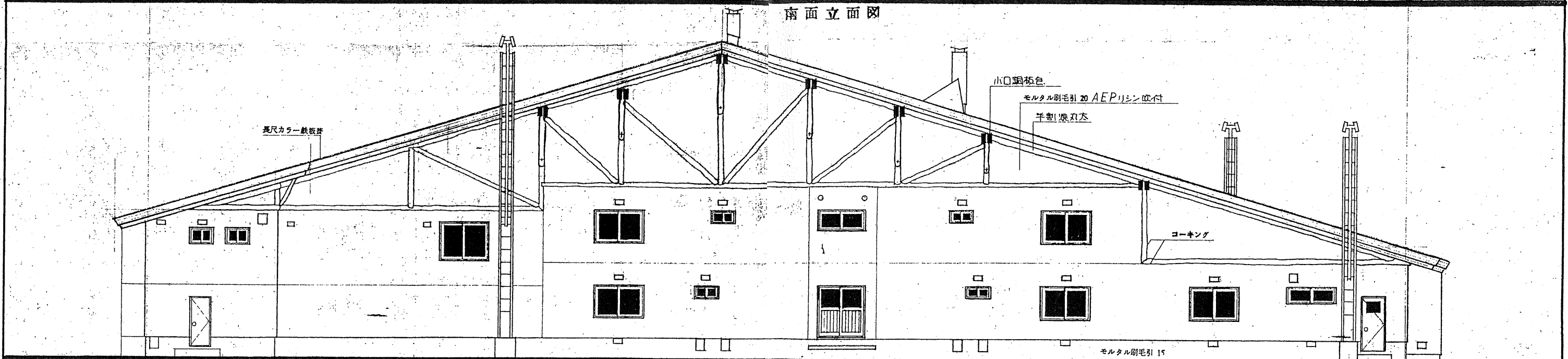
北面立面図
