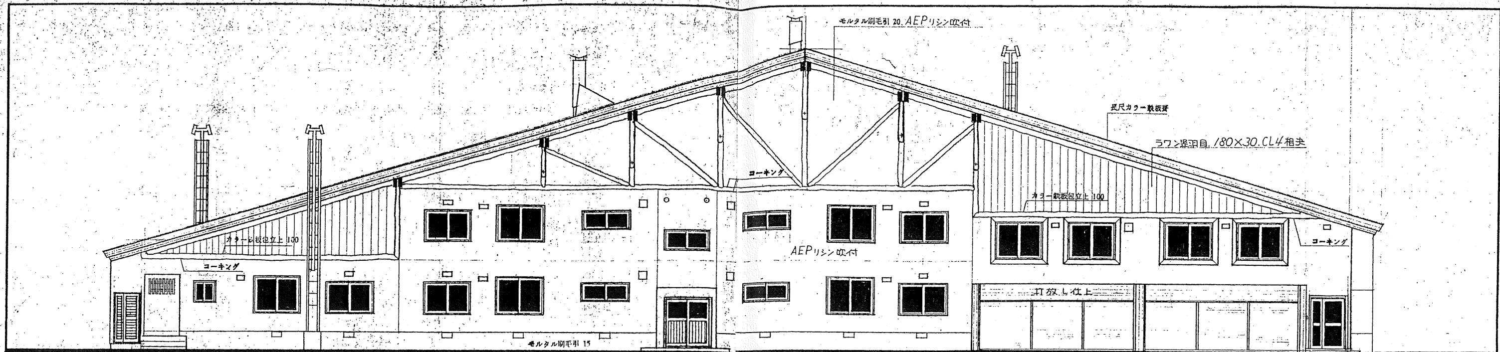
南面立面図
