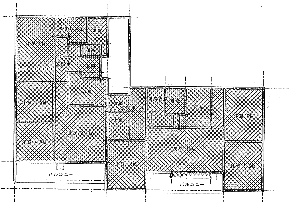
小屋断熱伏図 S=1/100
