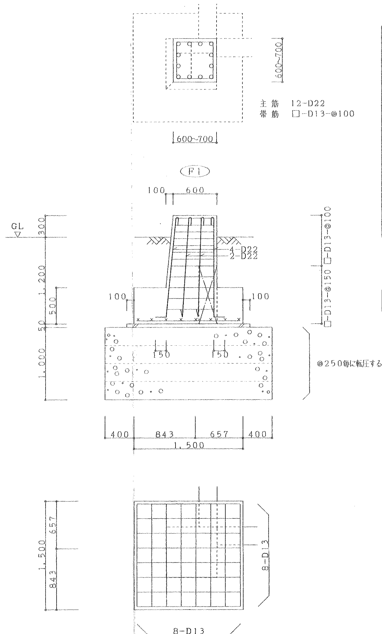
基礎リスト S1:30
