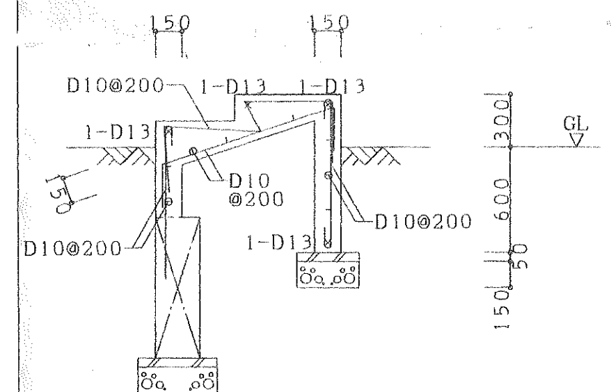
下り壁W15 S1:30
